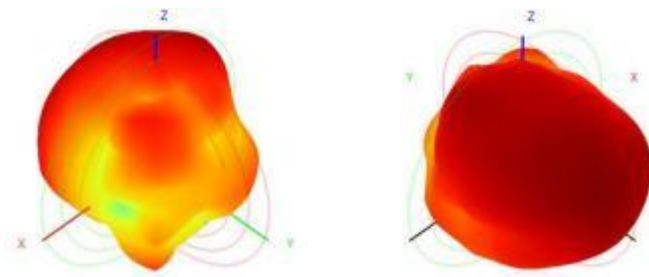
E2 (yz)
