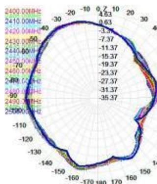
E1 (xz)
