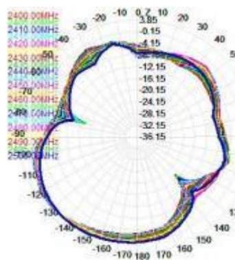
E1( XZ)
