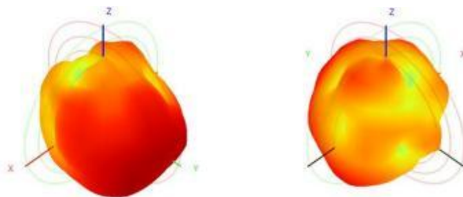
E2 (YZ)
