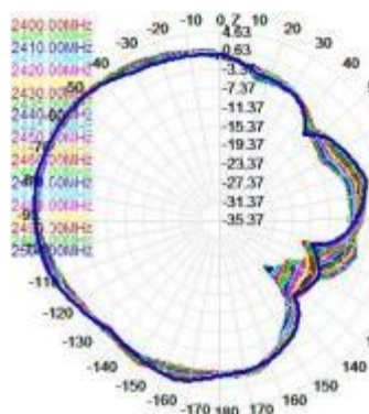
E2 (yz)
