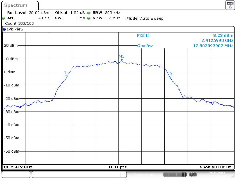
11G_Ant1_2412
