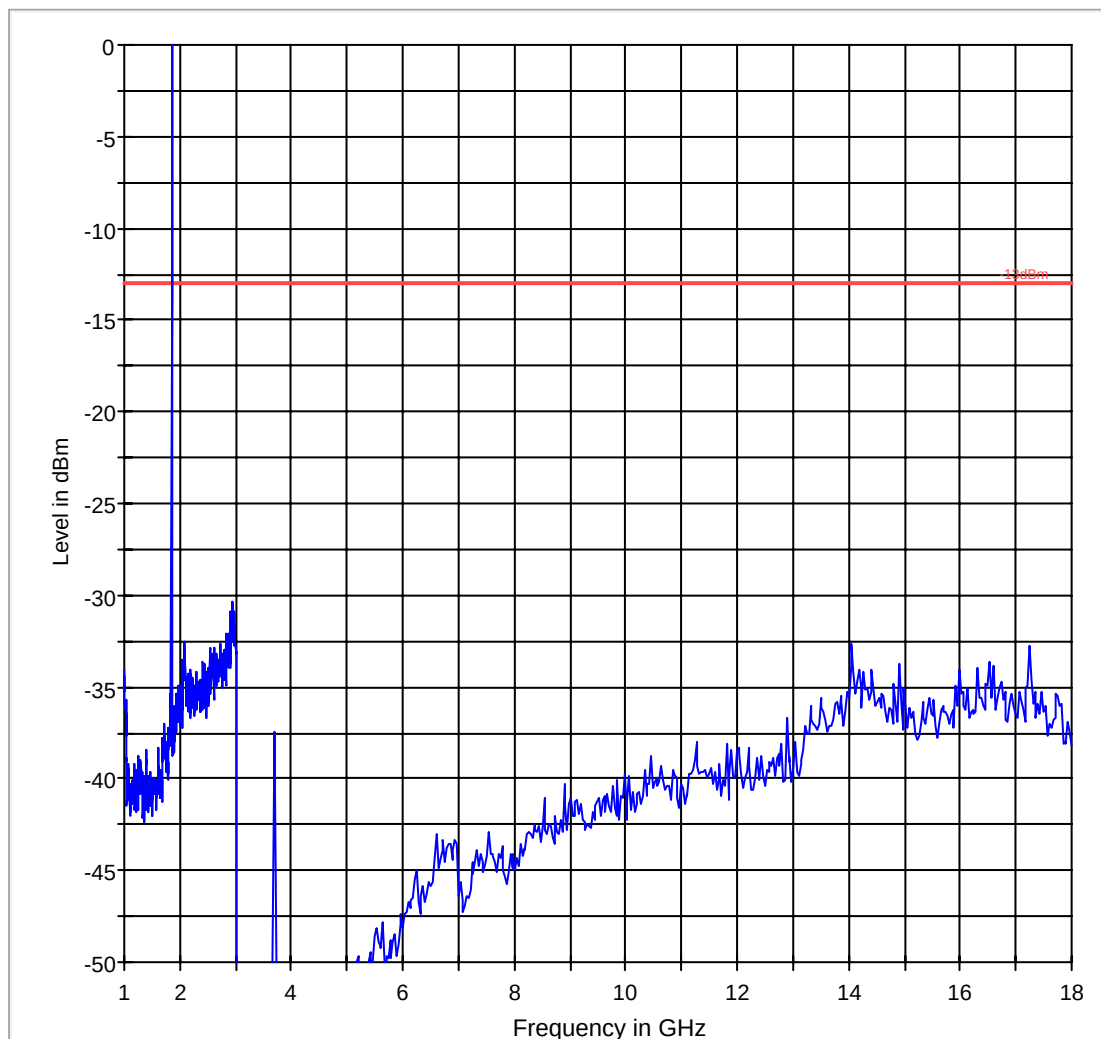
FCC 24 1-18GHz
