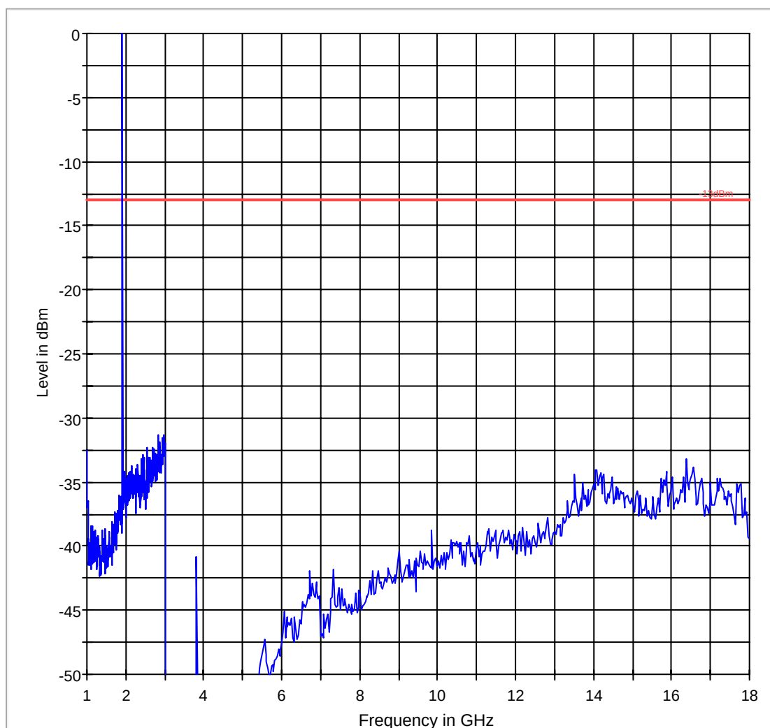
FCC 24 1-18GHz
