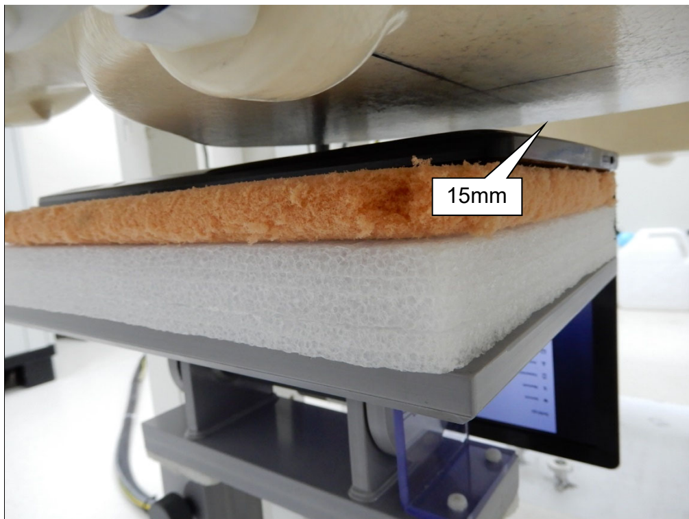
EUT Bottom_WWAN_15mm
