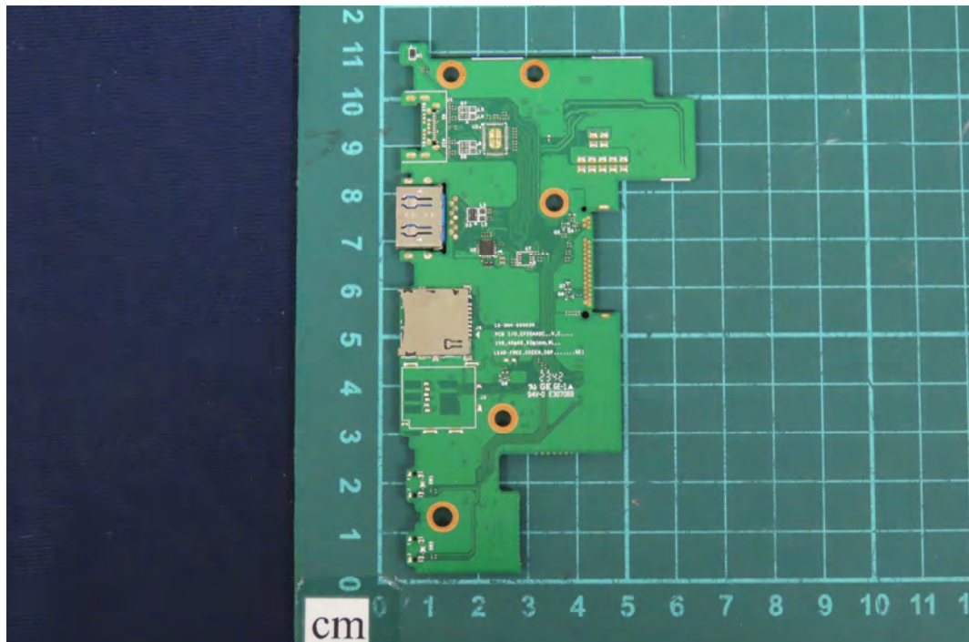
(18) EUT Photo
