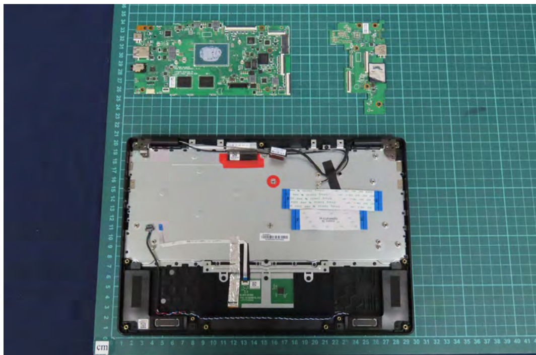
(12) EUT Photo
