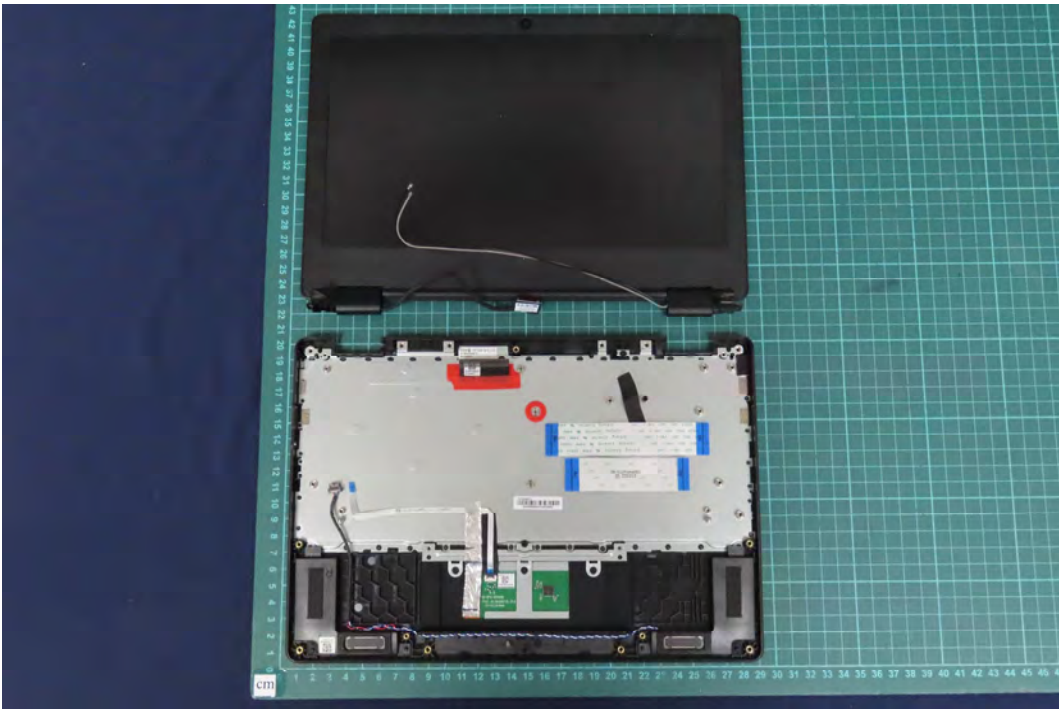
(24) EUT Photo
