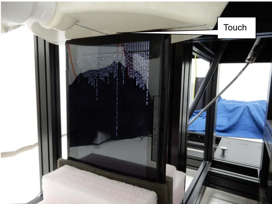
EUT Left-side(PAD)
