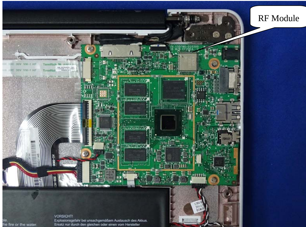
(9) EUT Photo
