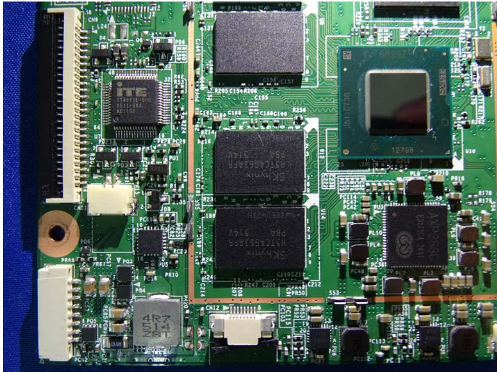
(19) EUT Photo
