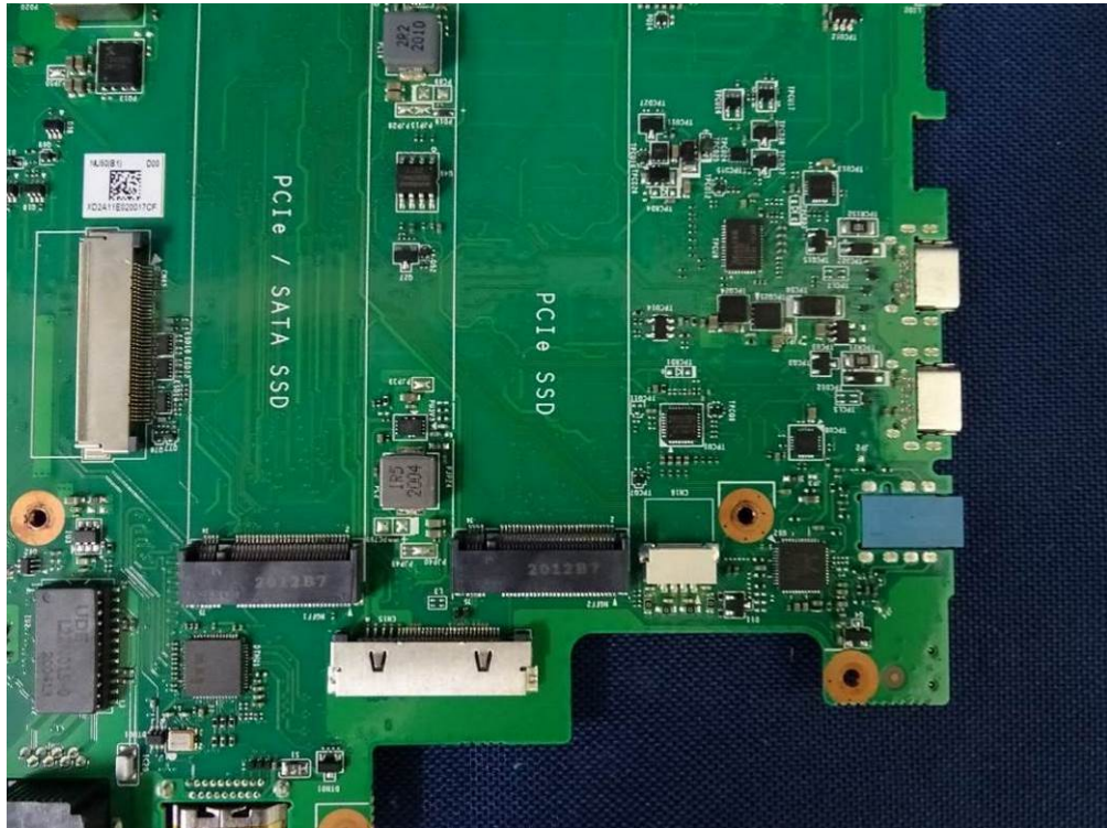
(31) EUT Photo
