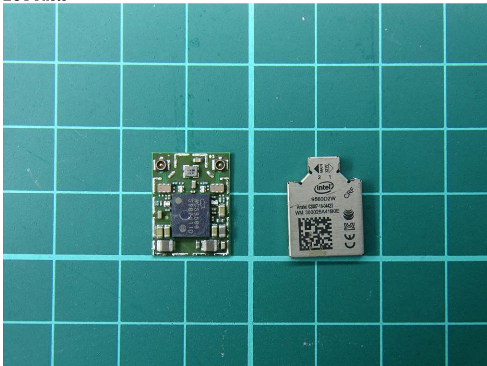
(49) EUT Photo
