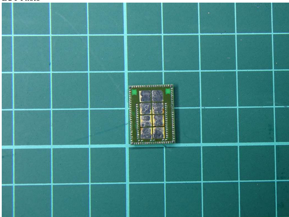
(48) EUT Photo
