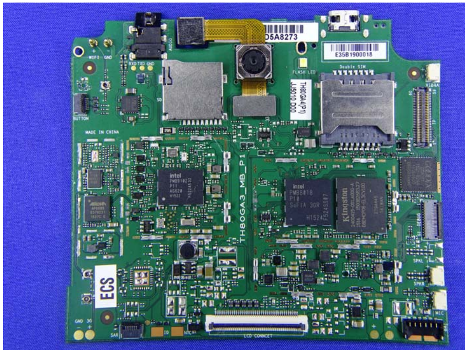
(6) EUT Photo
