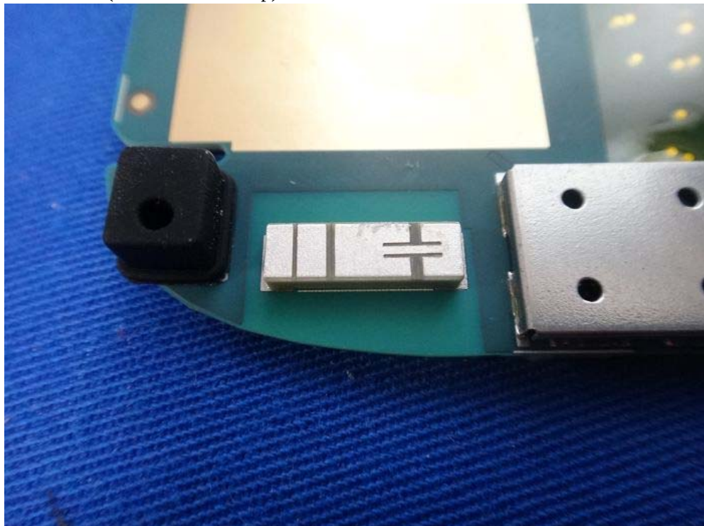
(14) EUT Photo (Aux Antenna-Chip)
