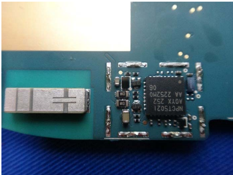
(12) EUT Photo
