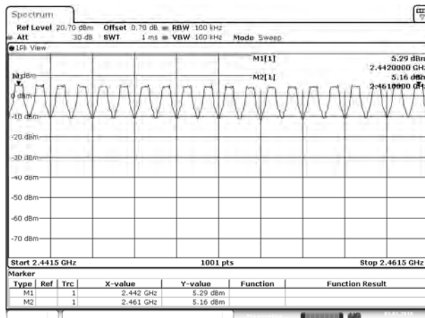
2442-2461MHz
