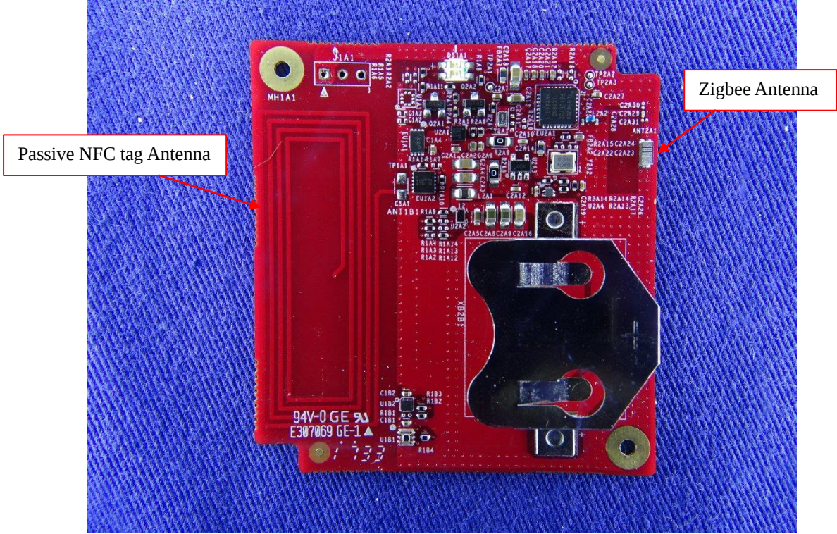
(6) EUT Photo
