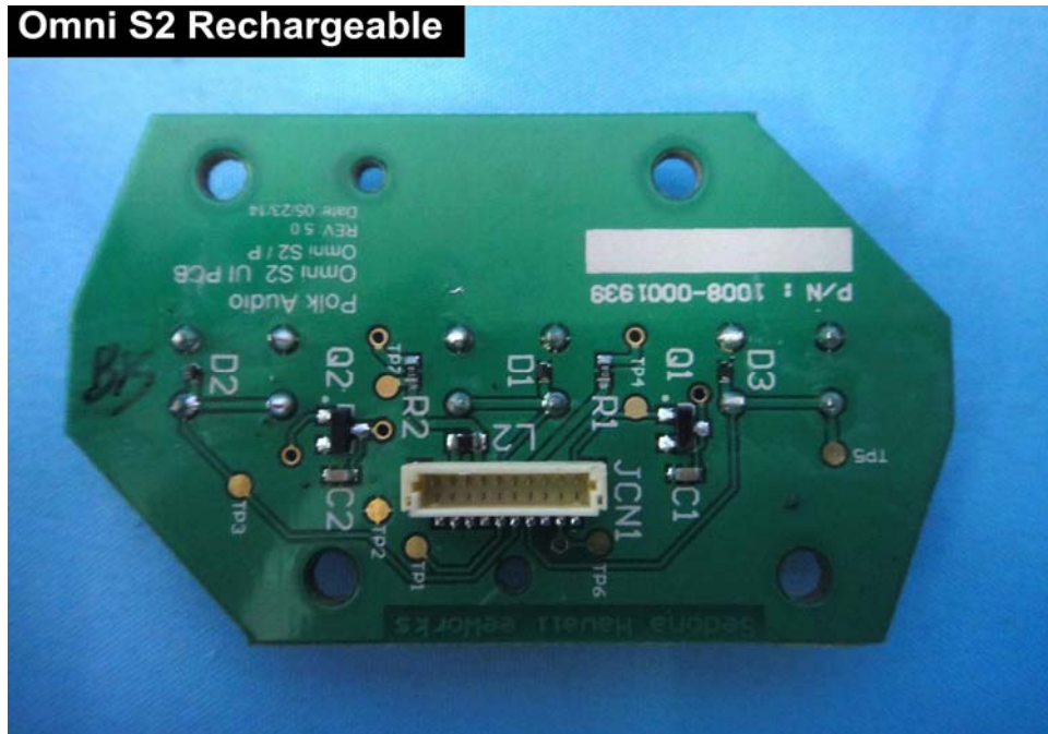
EUT Photo 22 )
