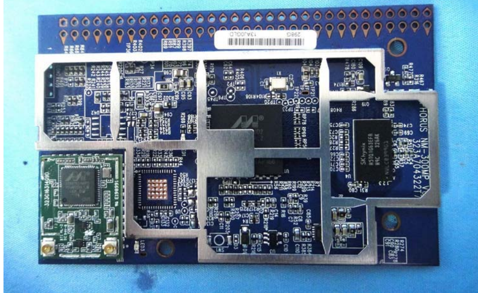
EUT Photo 34 )
