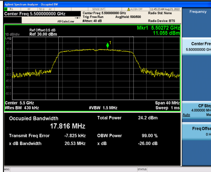
11N20MIMO_Ant2_5500
