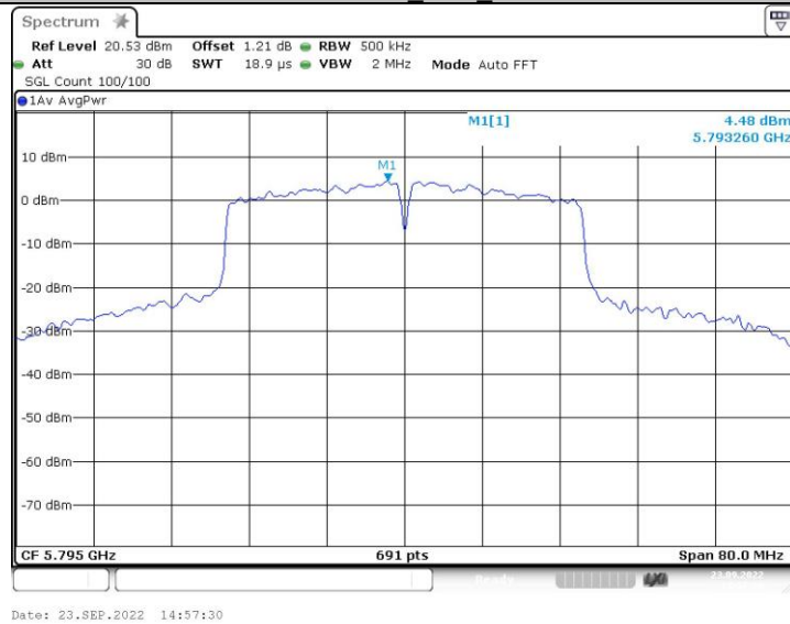
11N40MIMO_Ant2_5795
