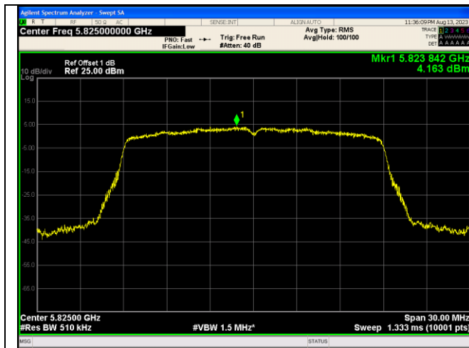
IEEE 802.11ac Channel 165 20MHz Antenna 2
