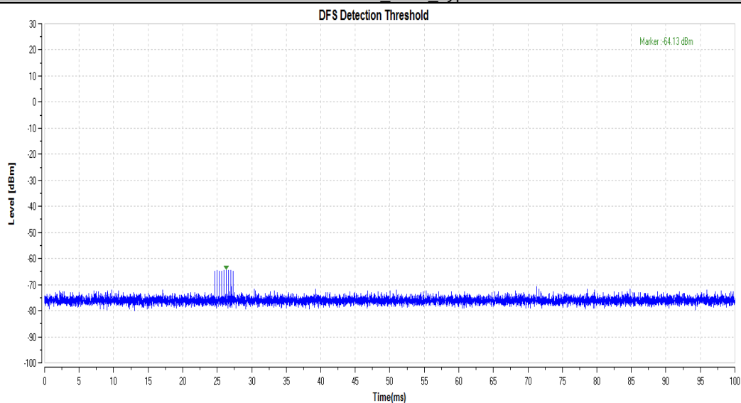
11AX160MIMO_5570_Type6
