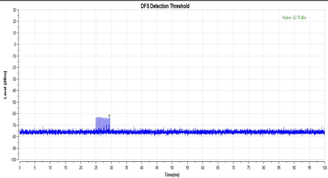
11AX160MIMO_5570_Type3
