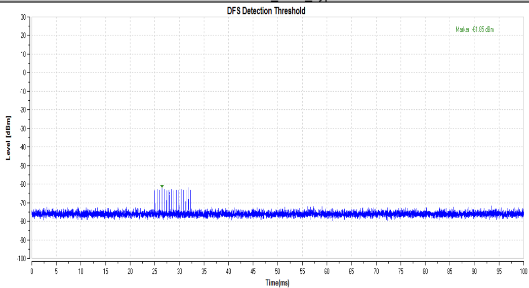
11AX160MIMO_5570_Type4
