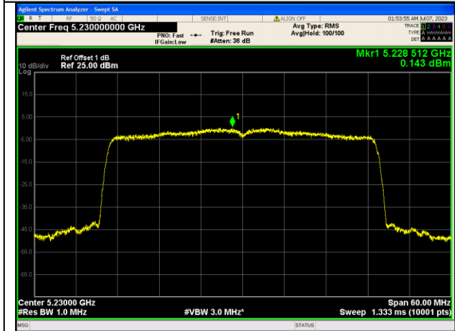
IEEE 802.11ax_Channel 46_40MHz_Antenna 0_RU&amp;Index 484RU65
