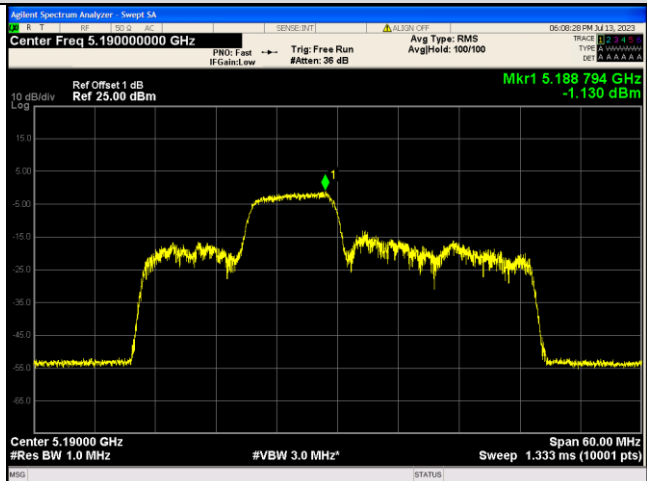
IEEE 802.11ax_Channel 38_40MHz_Antenna 0_RU&amp;Index 106RU54
