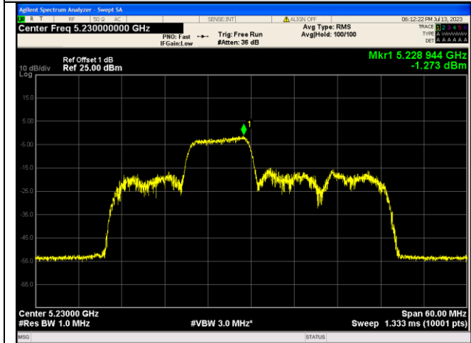
IEEE 802.11ax_Channel 46_40MHz_Antenna 0_RU&amp;Index 106RU54
