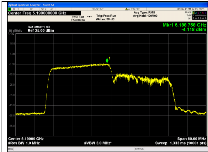
IEEE 802.11ax_Channel 38_40MHz_Antenna 0_RU&amp;Index 242RU61
