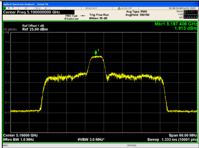
IEEE 802.11ax_Channel 38_40MHz_Antenna 0_RU&amp;Index 52RU40
