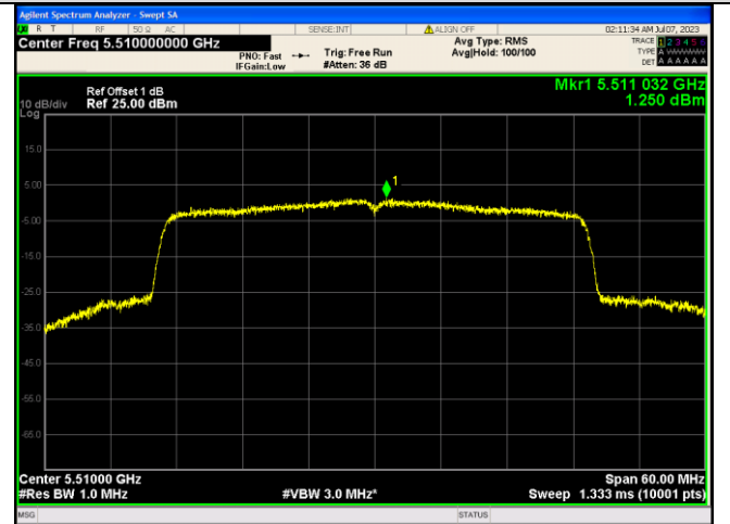
IEEE 802.11ax_Channel 102_40MHz_Antenna 1_RU&amp;Index 484RU65
