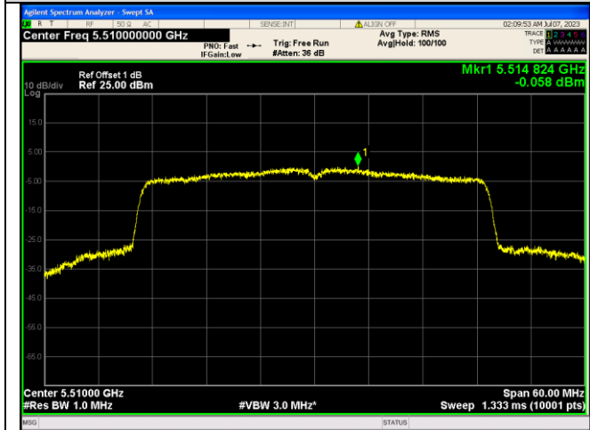
IEEE 802.11ax_Channel 102_40MHz_Antenna 0_RU&amp;Index 484RU65
