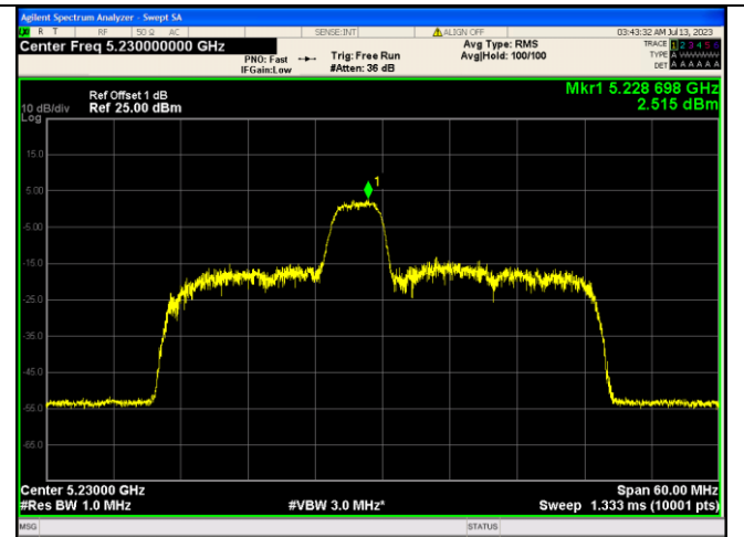
IEEE 802.11ax_Channel 46_40MHz_Antenna 1_RU&amp;Index 52RU40
