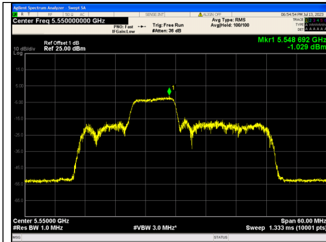
IEEE 802.11ax Channel 110_40MHz_Antenna 0 RU&Index 106RU54
