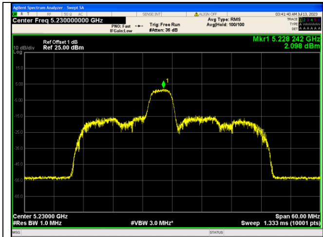
IEEE 802.11ax_Channel 46_40MHz_Antenna 0_RU&amp;Index 52RU40
