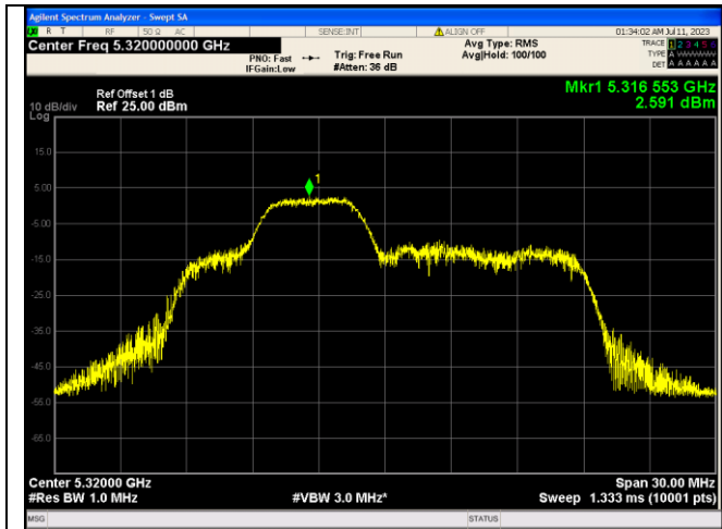
IEEE 802.11ax_Channel 64_20MHz_Antenna 0_RU&amp;Index 52RU38
