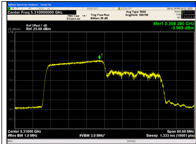
IEEE 802.11ax_Channel 62_40MHz_Antenna 0_RU&amp;Index 242RU61
