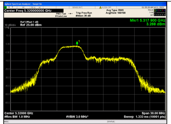
IEEE 802.11ax_Channel 64_20MHz_Antenna 1_RU&amp;Index 52RU38
