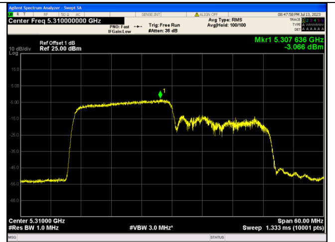
IEEE 802.11ax_Channel 62_40MHz_Antenna 1_RU&amp;Index 242RU61
