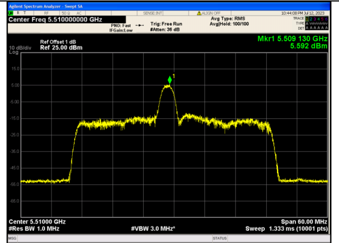
IEEE 802.11ax_Channel 102_40MHz_Antenna 1_RU&amp;Index 26RU8
