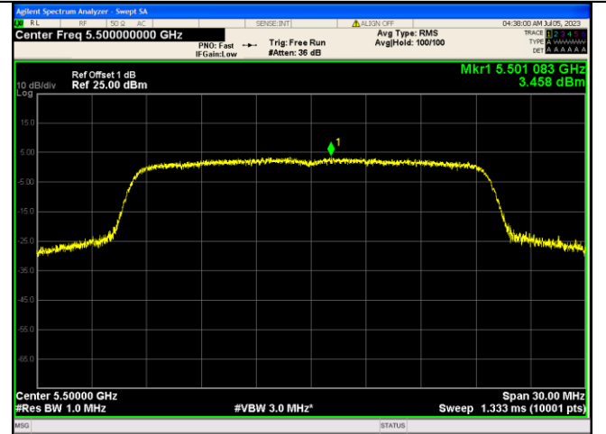
IEEE 802.11ax_Channel 100_20MHz_Antenna 1_RU&amp;Index 242RU61
