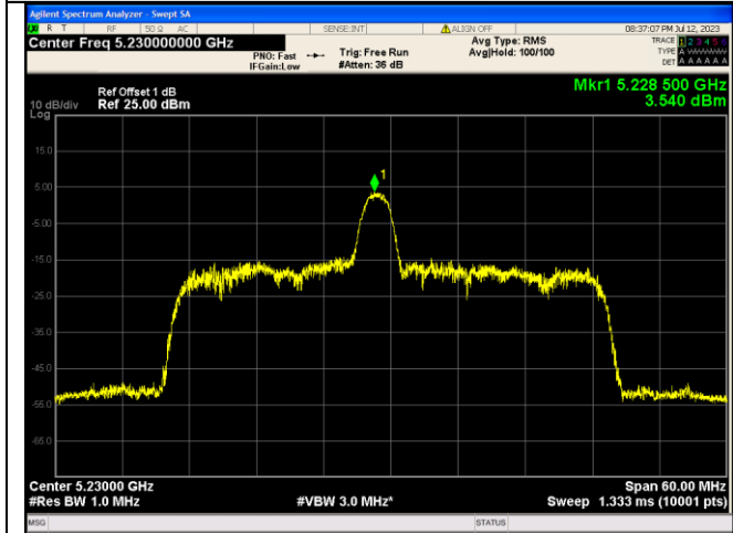
IEEE 802.11ax_Channel 46_40MHz_Antenna 0_RU&amp;Index 26RU8
