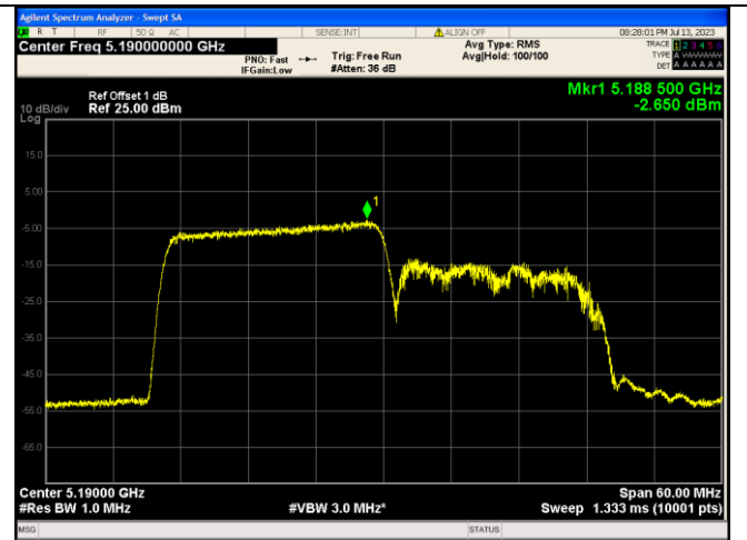
IEEE 802.11ax_Channel 38_40MHz_Antenna 1_RU&amp;Index 242RU61
