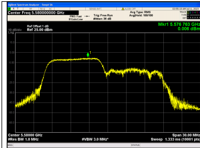
IEEE 802.11ax Channel 116_20MHz_Antenna 0 RU&Index 106RU53
