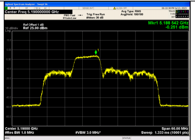
IEEE 802.11ax_Channel 38_40MHz_Antenna 1_RU&amp;Index 106RU54
