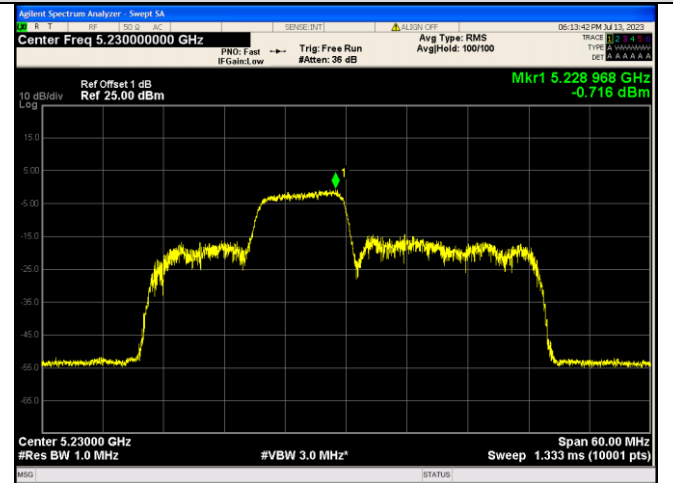
IEEE 802.11ax_Channel 46_40MHz_Antenna 1_RU&amp;Index 106RU54
