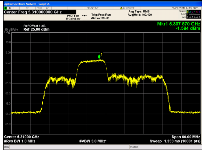
IEEE 802.11ax_Channel 62_40MHz_Antenna 0_RU&amp;Index 106RU54
