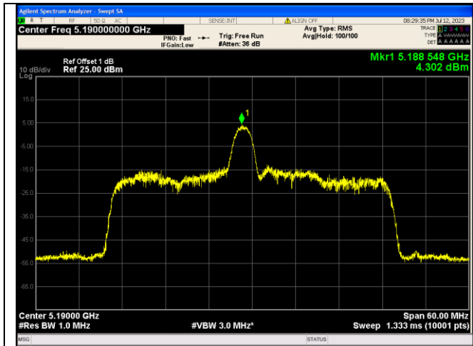
IEEE 802.11ax_Channel 38_40MHz_Antenna 0_RU&amp;Index 26RU8
