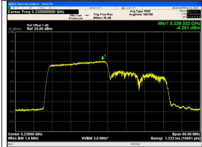
IEEE 802.11ax_Channel 46_40MHz_Antenna 0_RU&amp;Index 242RU61
