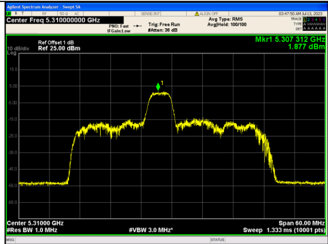
IEEE 802.11ax_Channel 62_40MHz_Antenna 0_RU&amp;Index 52RU40
