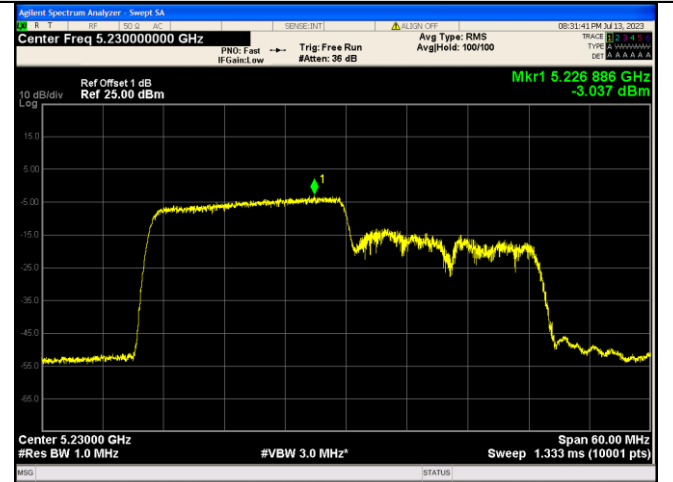
IEEE 802.11ax_Channel 46_40MHz_Antenna 1_RU&amp;Index 242RU61
