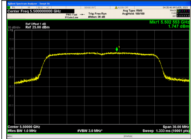
IEEE 802.11ax_Channel 100_20MHz_Antenna 0_RU&amp;Index 242RU61
