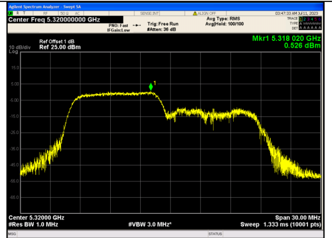
IEEE 802.11ax_Channel 64_20MHz_Antenna 1_RU&amp;Index 106RU53
