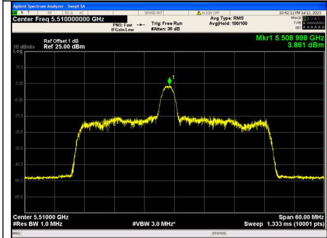
IEEE 802.11ax_Channel 102_40MHz_Antenna 0_RU&amp;Index 26RU8
