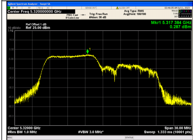
IEEE 802.11ax_Channel 64_20MHz_Antenna 0_RU&amp;Index 106RU53
