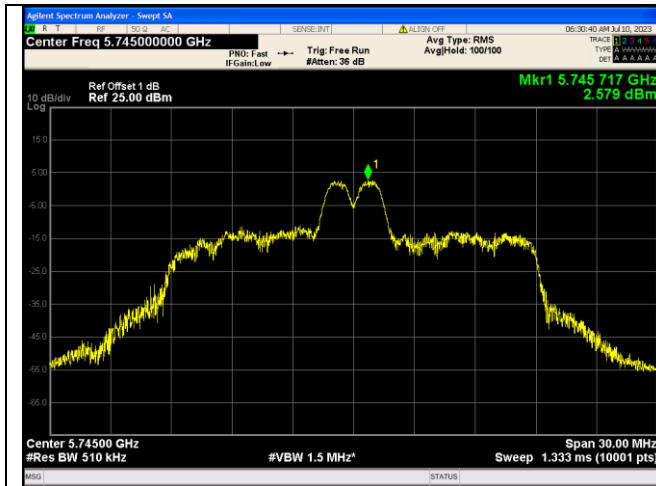
IEEE 802.11ax_Channel 149_20MHz_Antenna 0_RU&Index 26RU4
