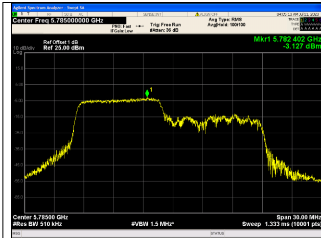
IEEE 802.11ax Channel 157 20MHz_Antenna 0 RU&Index 106RU53
