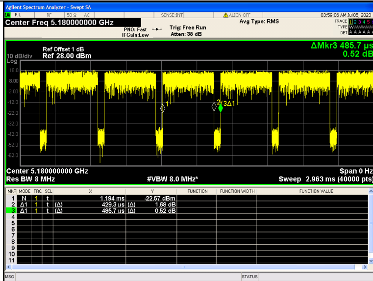
IEEE 802.11ax 20MHz Channel 36
