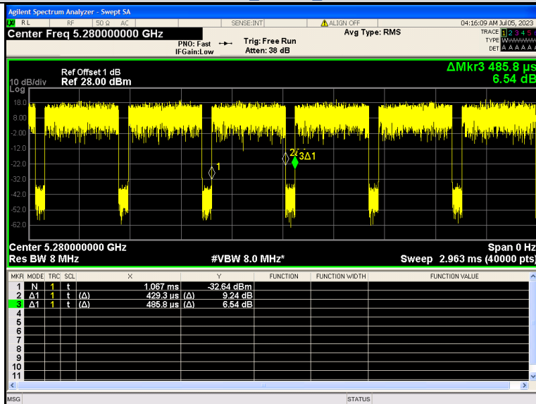
IEEE 802.11ax 20MHz Channel 56
