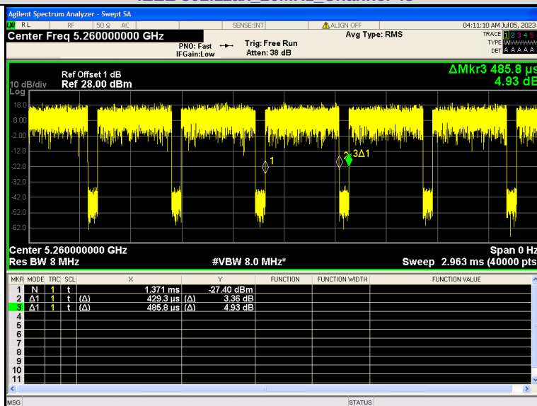
IEEE 802.11ax 20MHz Channel 52
