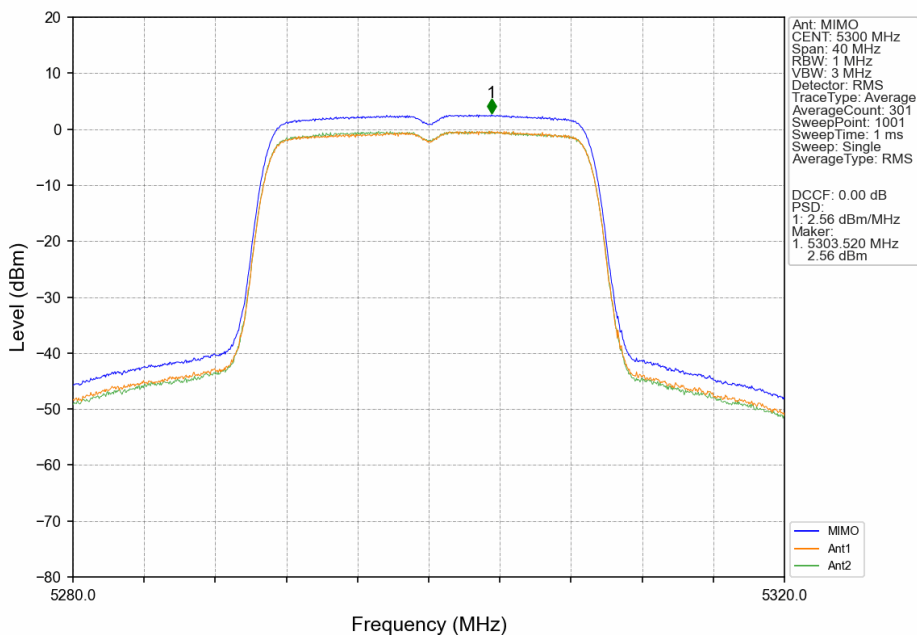
802.11n(HT20)_MCH_5300MHz_MIMO_NTNV
