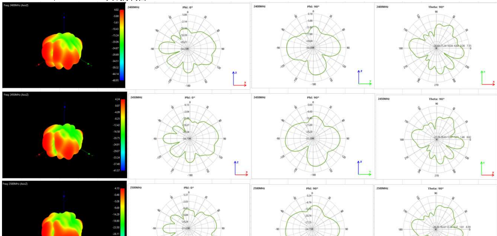
WIFI2.4G /5.8G L=428MM天线方向图
