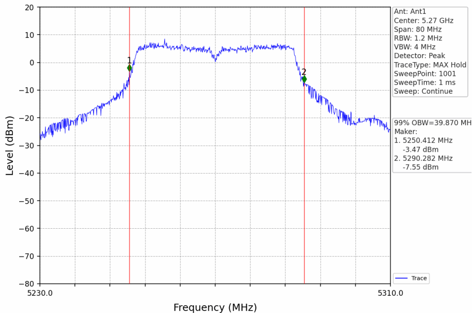
802.11ac(VHT40)_LCH_5270MHz_Ant1_NTNV
