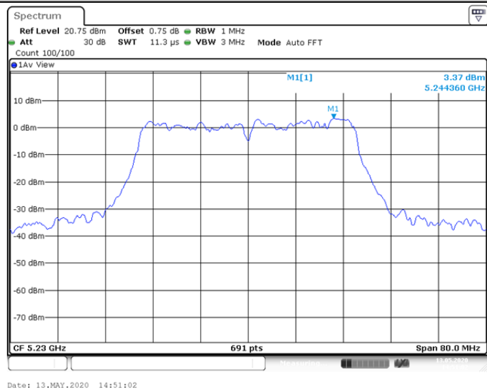
11N40SISO_Ant2_5230
