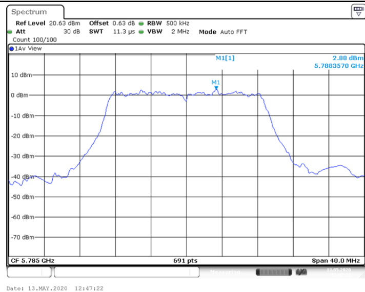
11N20SISO_Ant2_5785
