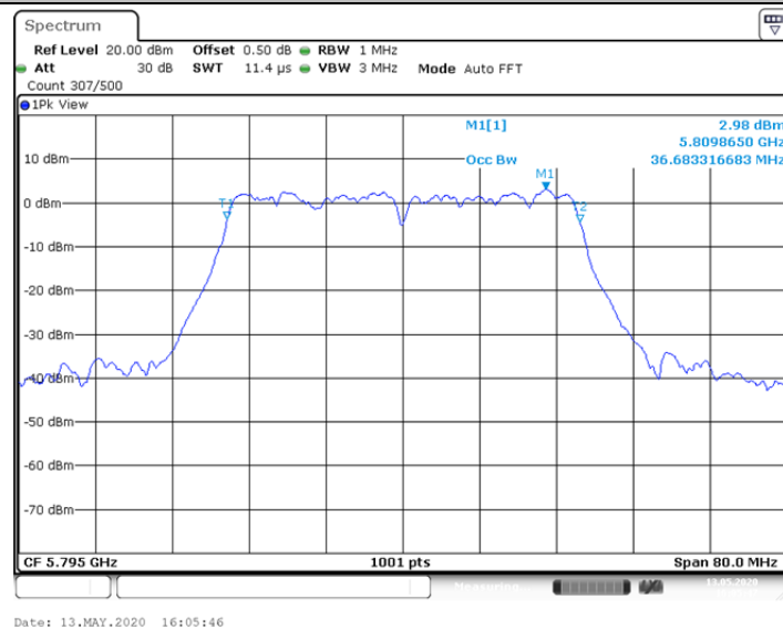
11AC40SISO_Ant2_5795
