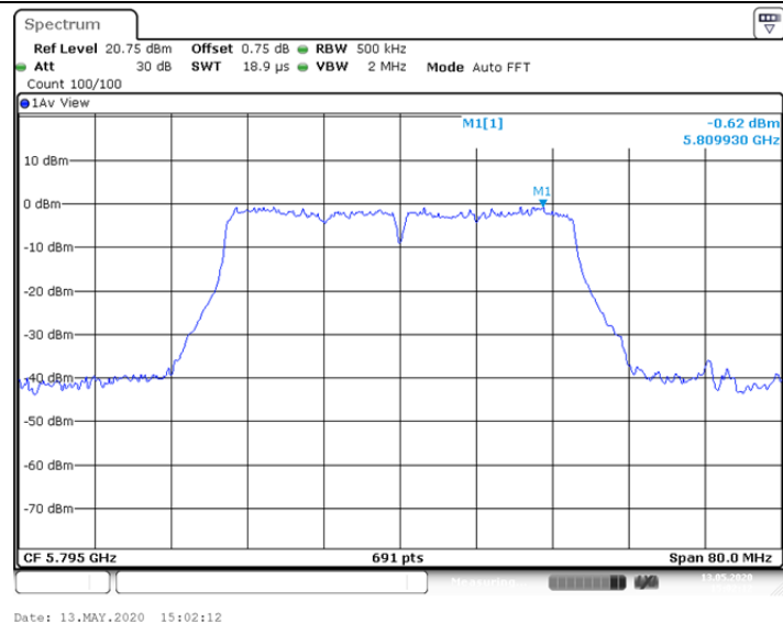
11N40SISO_Ant2_5795
