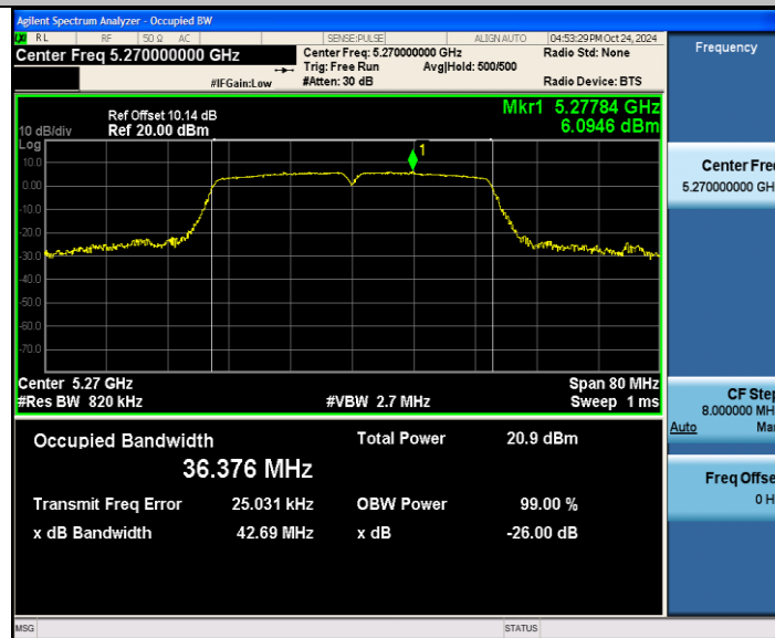
11AC40MIMO_Ant2_5270
