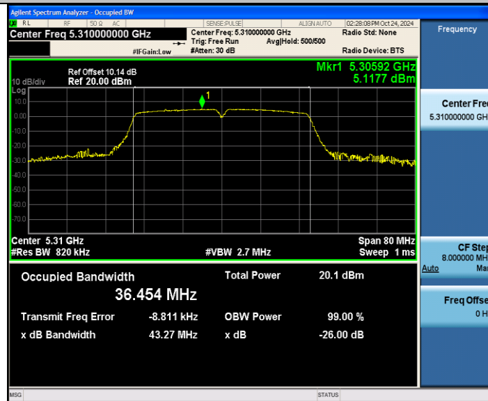
11N40MIMO_Ant2_5310
