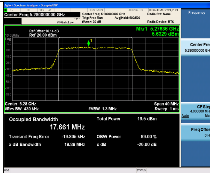
11AC20MIMO_Ant2_5280
