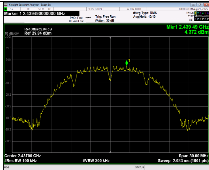
11B_Ant1_2437_30~1000
