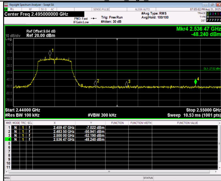
11N20MIMO_Ant2_High_2462
