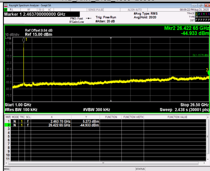
11B_Ant2_2462_0~Reference
