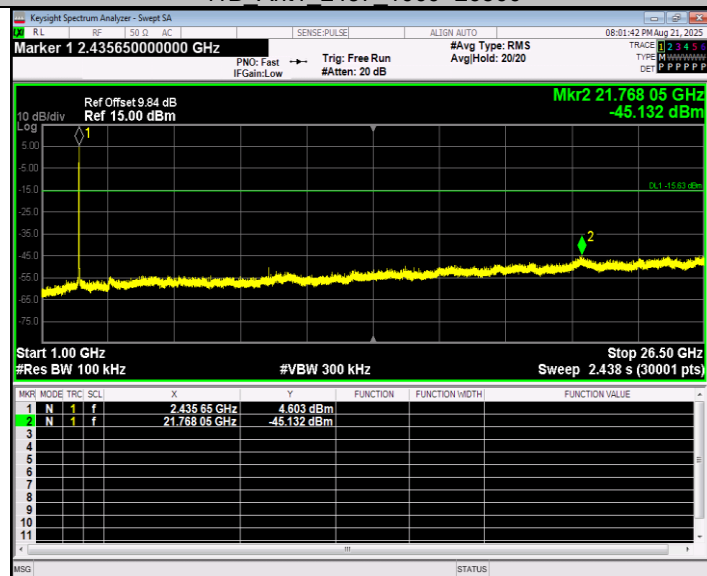
11B_Ant2_2437_0~Reference
