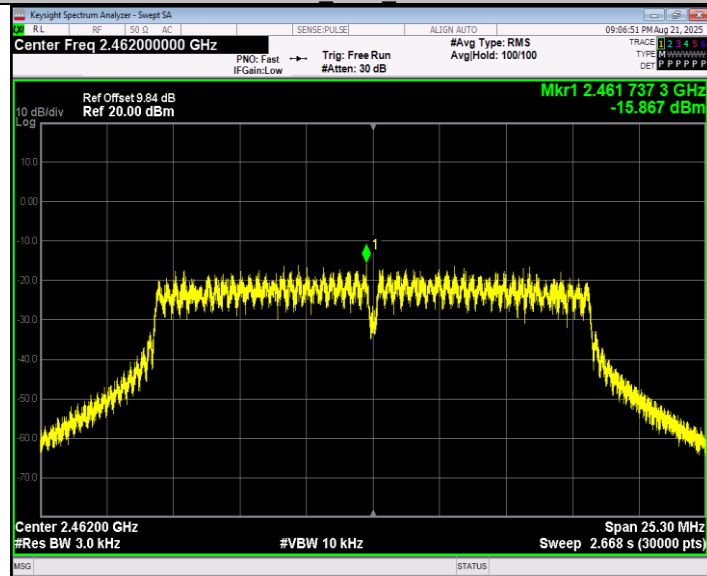
11G_Ant2_2462
