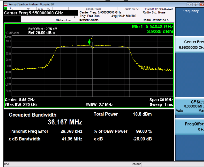
11N40MIMO_Ant2_5550
