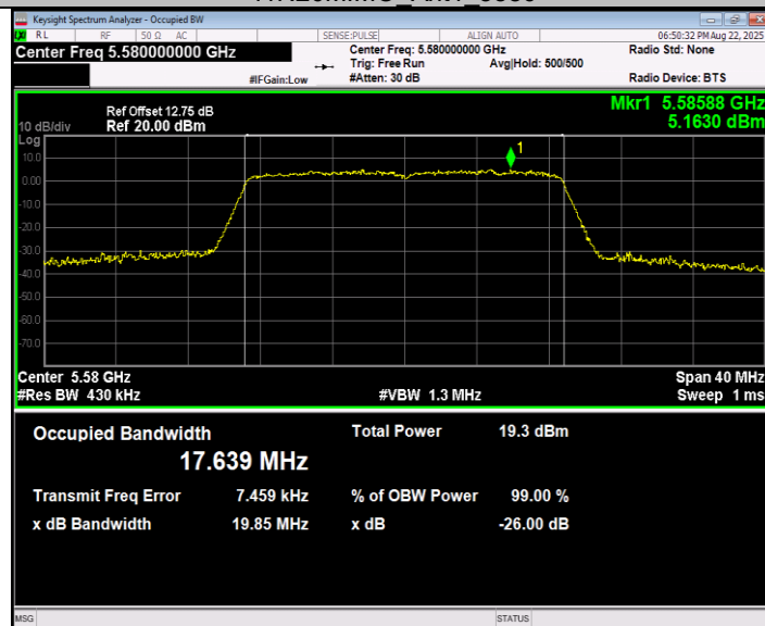
11N20MIMO_Ant2_5580
