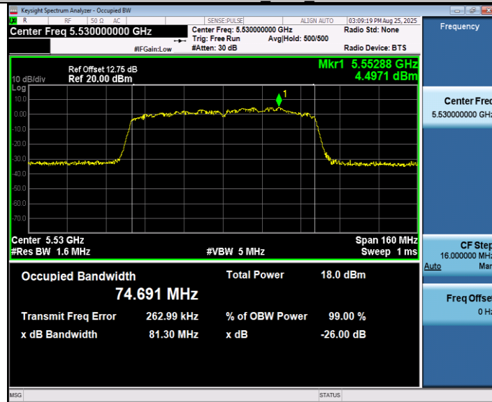
11AC80MIMO_Ant2_5530
