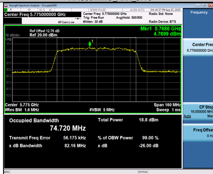
11AC80MIMO_Ant2_5775
