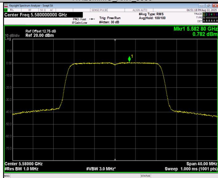
11N20MIMO_Ant2_5580
