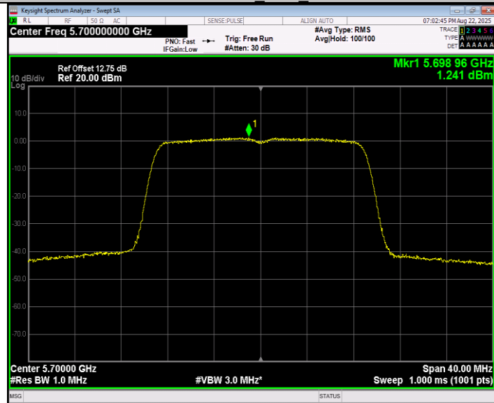
11N20MIMO_Ant2_5700
