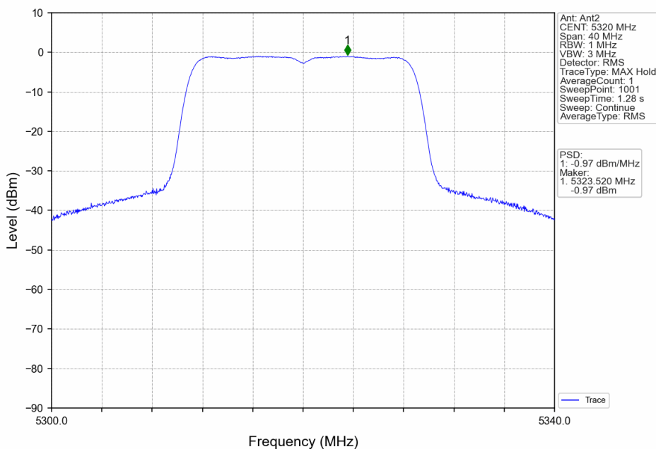
802.11n(HT20)_HCH_5320MHz_MIMO_NTNV
