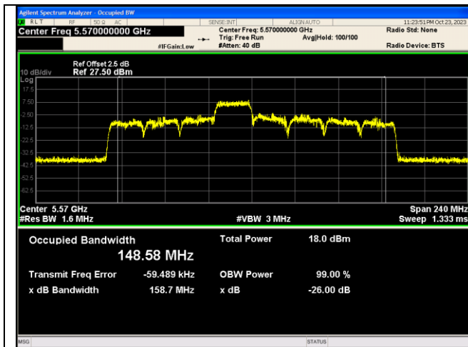
IEEE 802.11ax_Channel 114_160MHz_Antenna 2_RU&Index 242RU64
