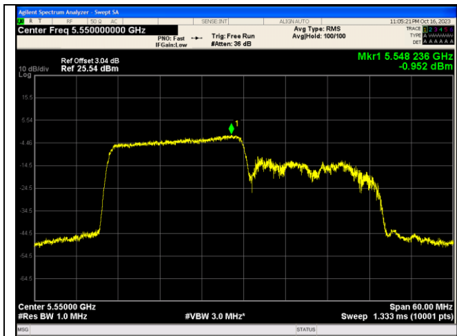
IEEE 802.11ax Channel 110 40MHz_Antenna 2 RU&Index 242RU61
