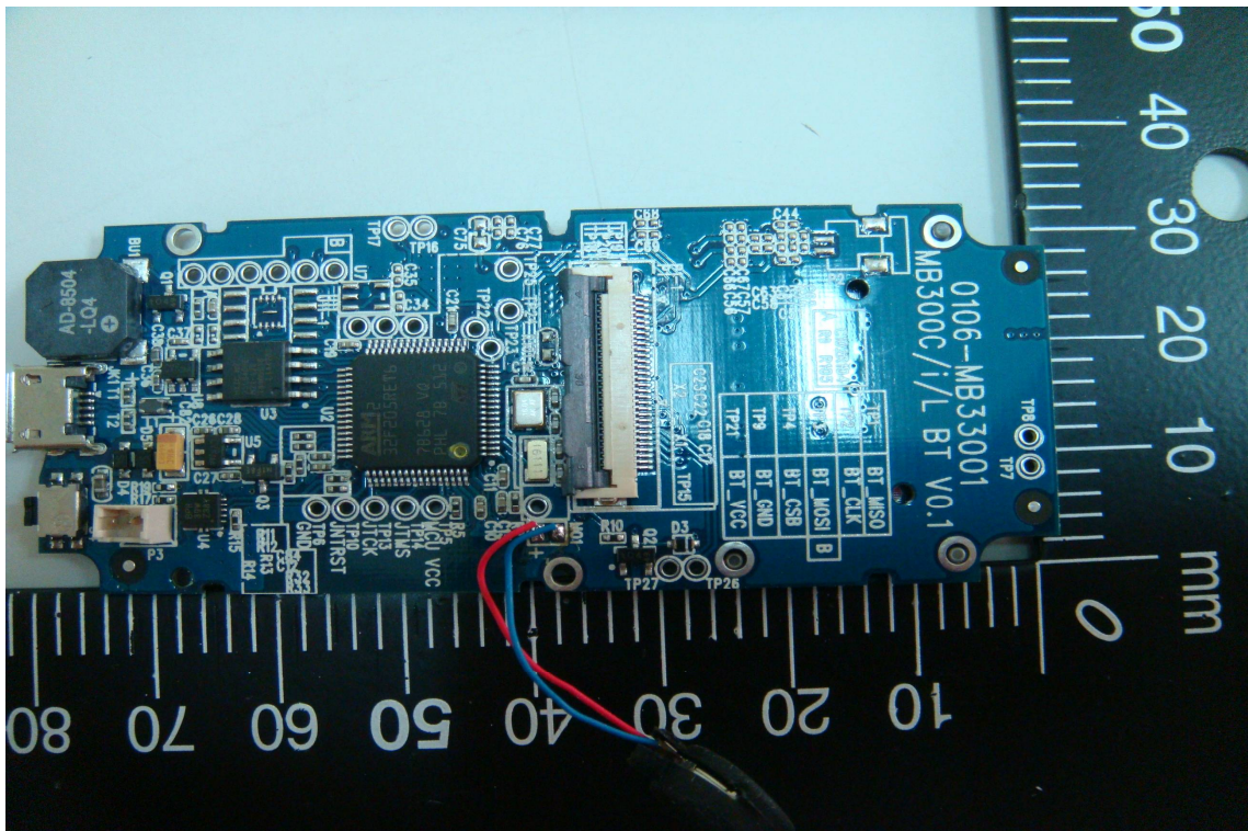
< PCB3-R >
