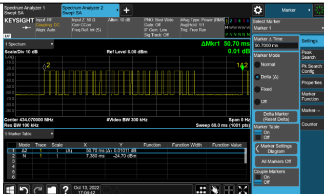
Ton 2 time
