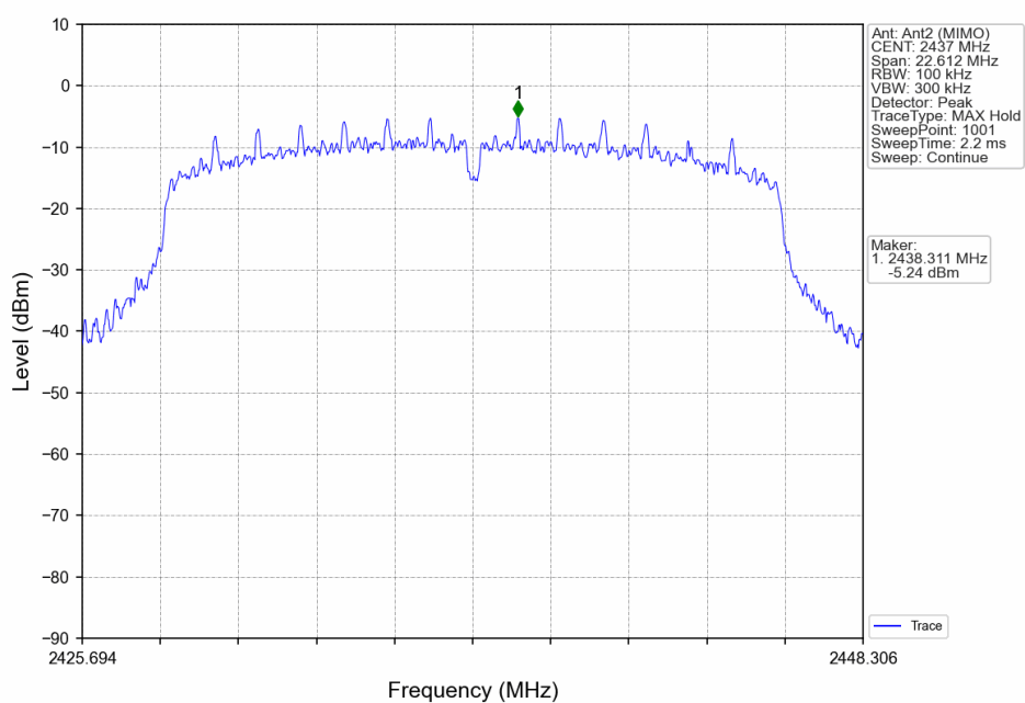
802.11n(HT20) MCH 2437MHz Ant2 (MIMO) NTN
