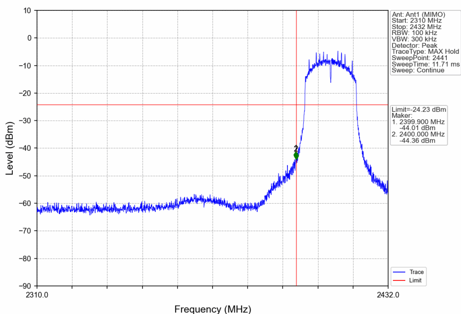
802.11n(HT20) LCH 2412MHz Ant1 (MIMO) NTV
