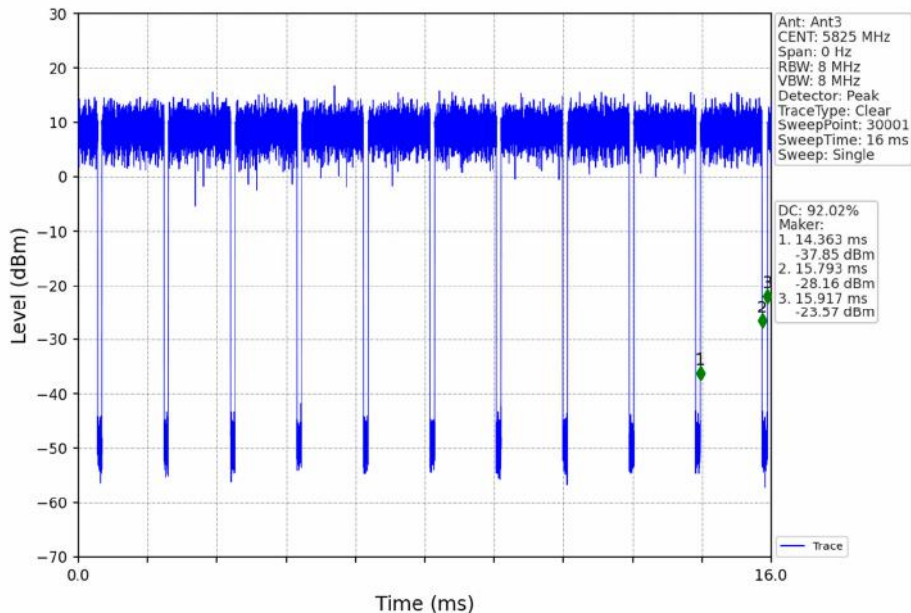
802.11a_HCH_5825MHz_Ant3_NTNV
