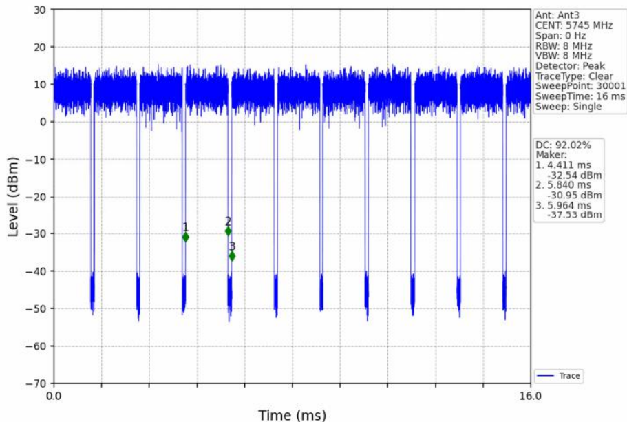
802.11a_LCH_5745MHz_Ant3_NTNV
