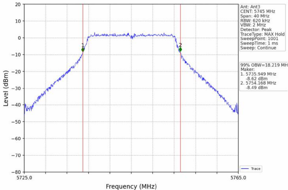
802.11a_LCH_5745MHz_Ant3_NTNV
