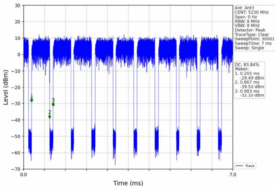
802.11n(HT40)_HCH_5230MHz_Ant3_NTNV
