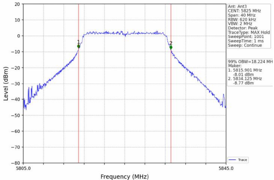
802.11a_HCH_5825MHz_Ant3_NTNV
