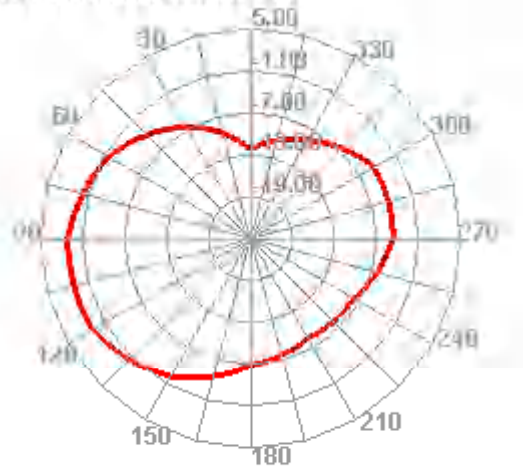
2450.000MHz H
