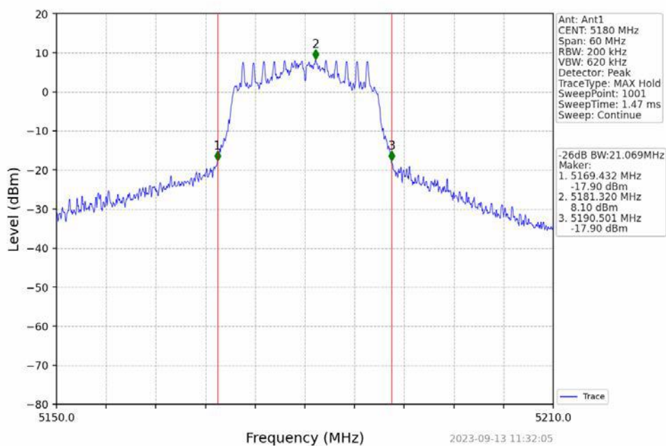
802.11n(HT20)_LCH_5180MHz_NTNV
