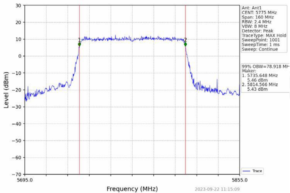
802.11ax(HEW80)_MCH_5775MHz_RU996_Left_NTNV
