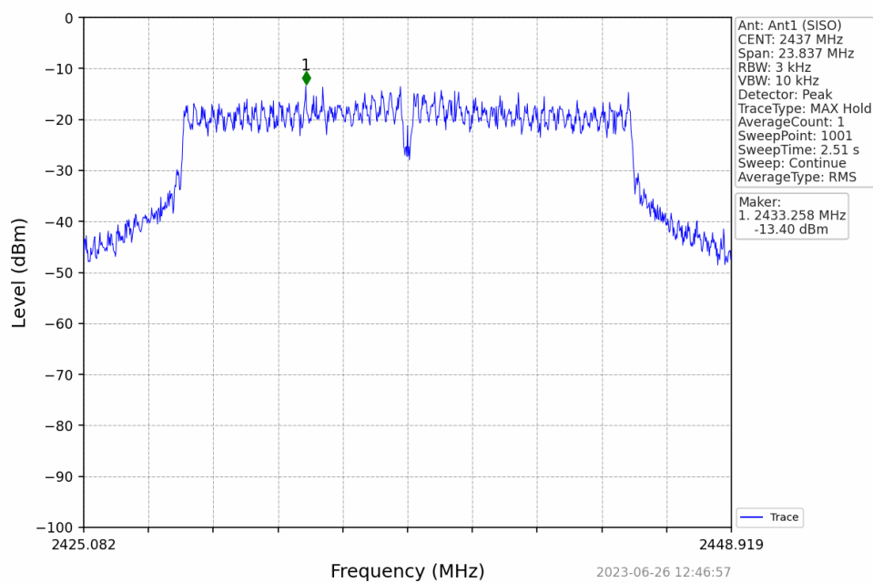
802.11g_MCH_2437MHz_Ant1 (SISO)_NTNV
