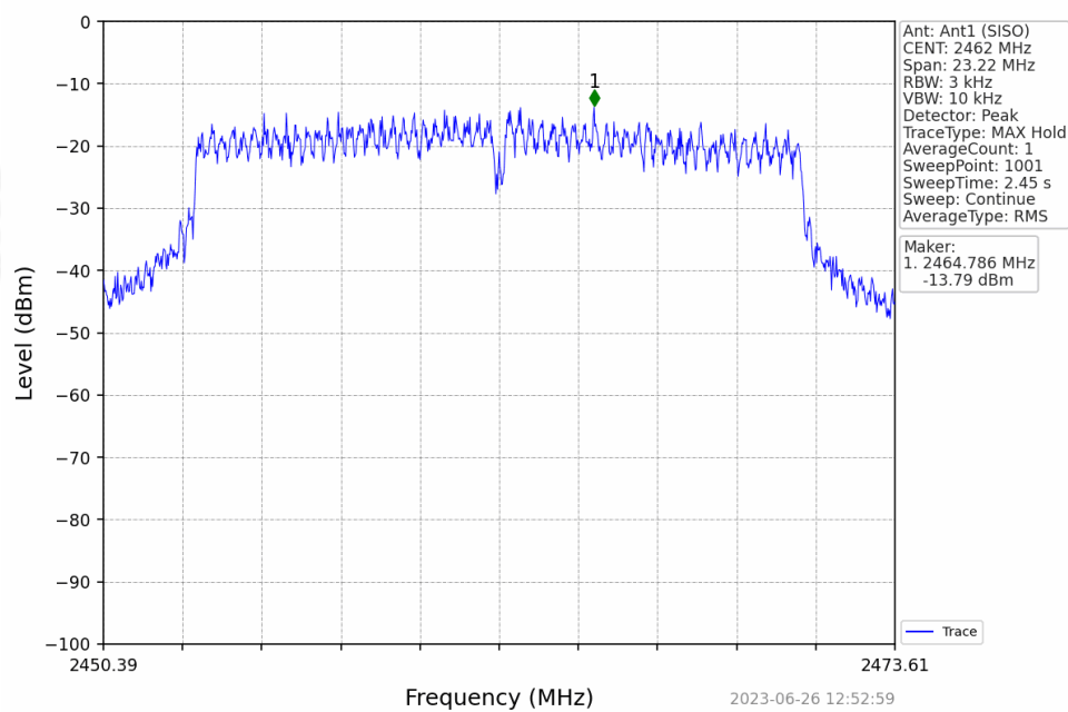
802.11n(HT20)_HCH_2462MHz_Ant1 (SISO)_NTNV
