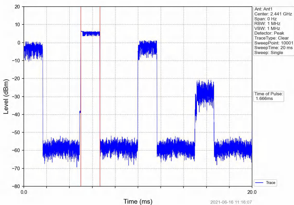
PI/4DQPSK_2DH3_HOPP_Ant1_NTNV
