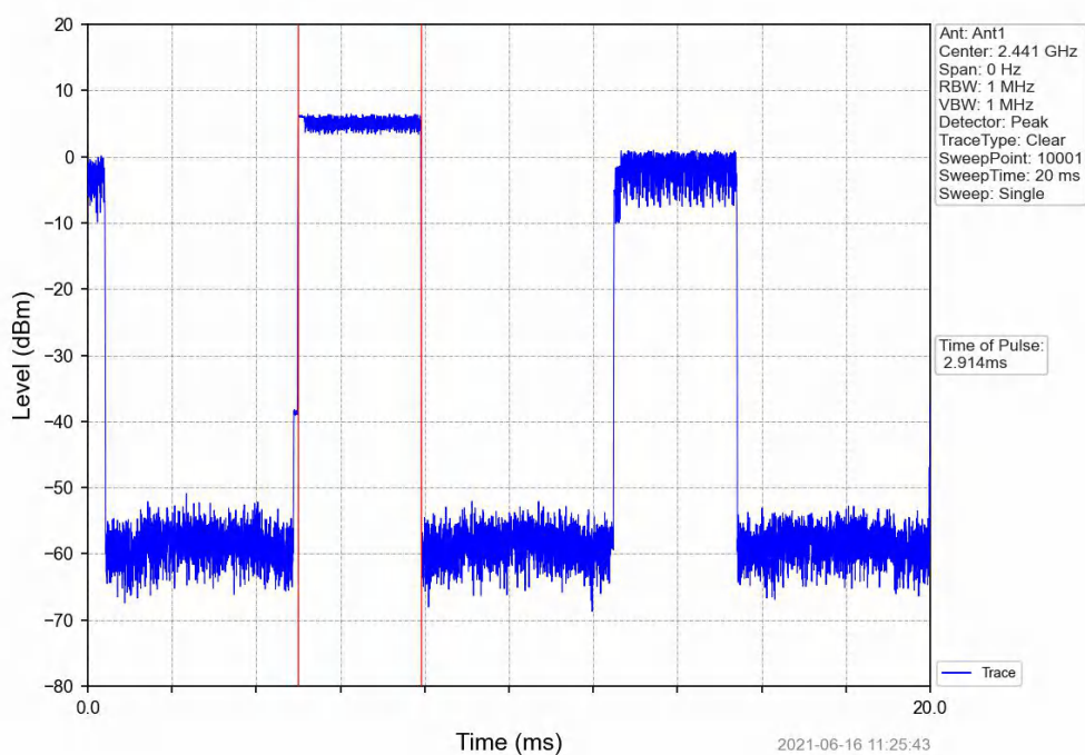
8DPSK 3DH5_HOPP_Ant1_NTNV
