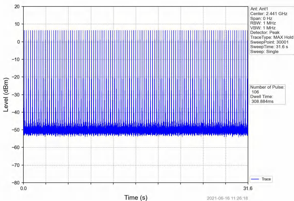
8DPSK 3DH5_HOPP_Ant1_NTNV
