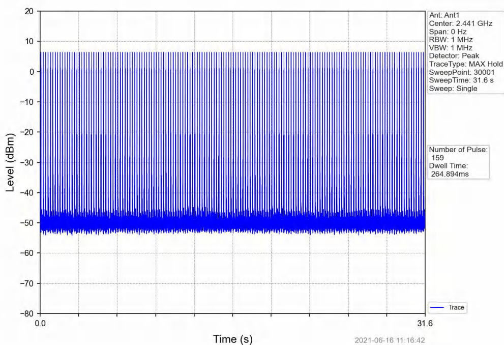
PI/4DQPSK_2DH3_HOPP_Ant1_NTNV
