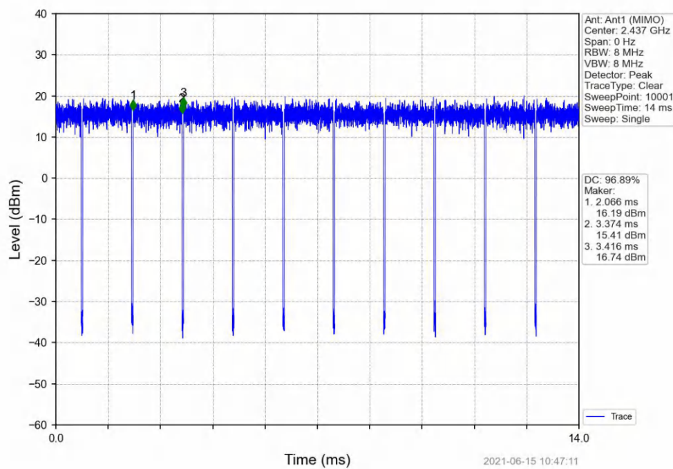
802.11n(HT20)_MCH_2437MHz_Ant1 (MIMO)_NTNV
