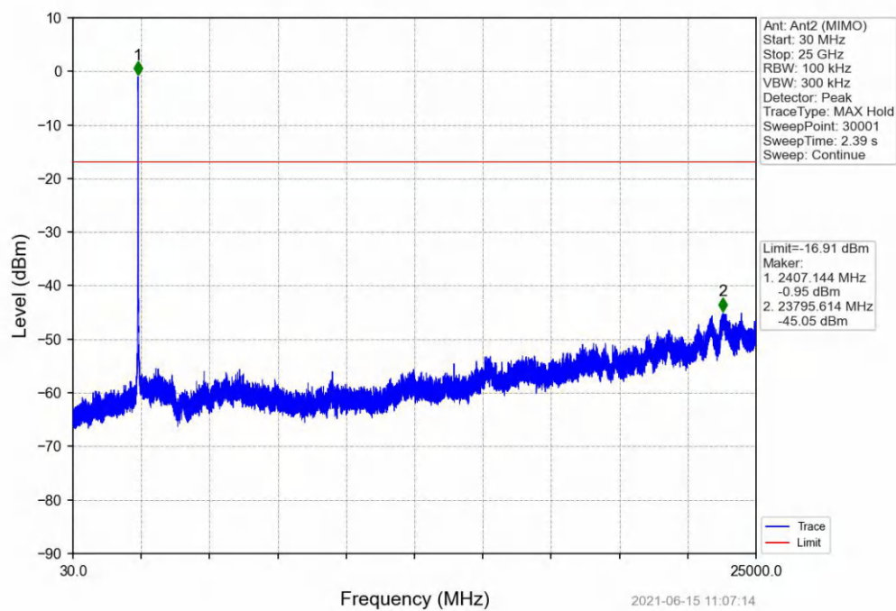
802.11n(HT20)_LCH_2412MHz_Ant2 (MIMO)_NTNV
