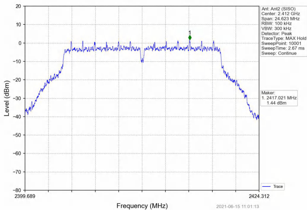
802.11g_LCH_2412MHz_Ant2 (SISO)_NTNV
