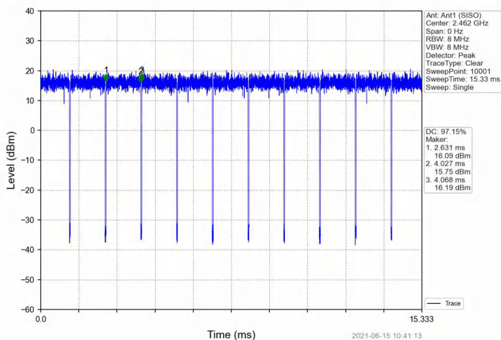
802.11g_HCH_2462MHz_Ant1 (SISO)_NTNV
