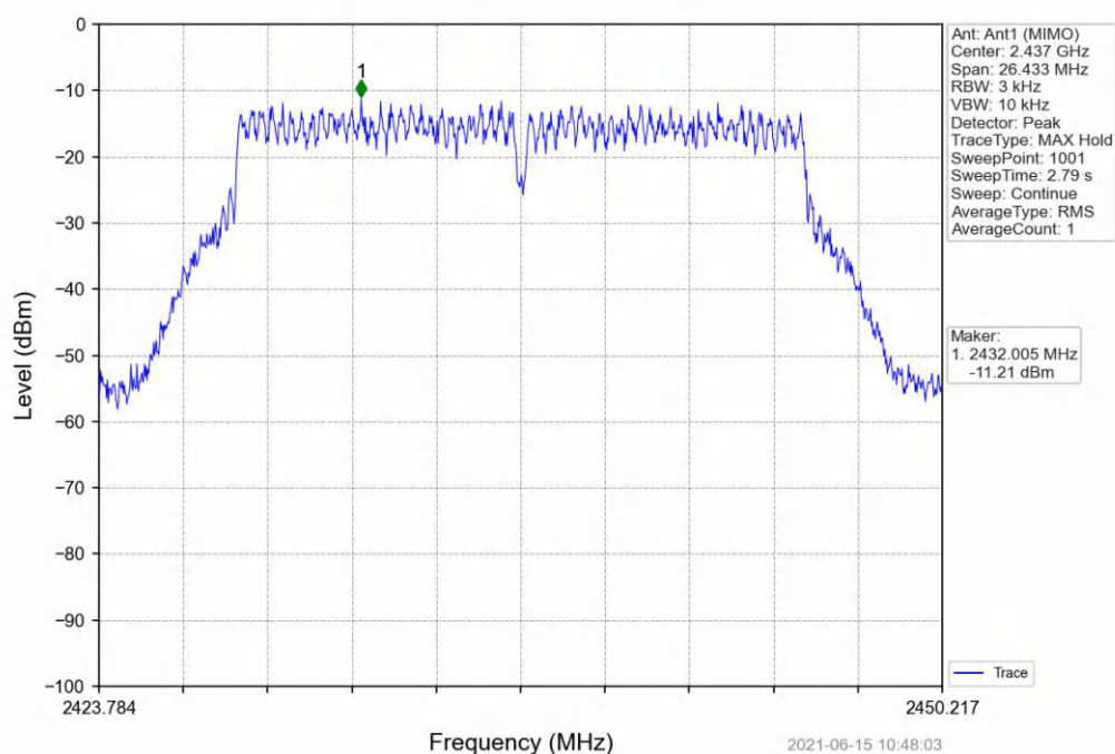
802.11n(HT20)_MCH_2437MHz_Ant1 (MIMO)_NTNV
