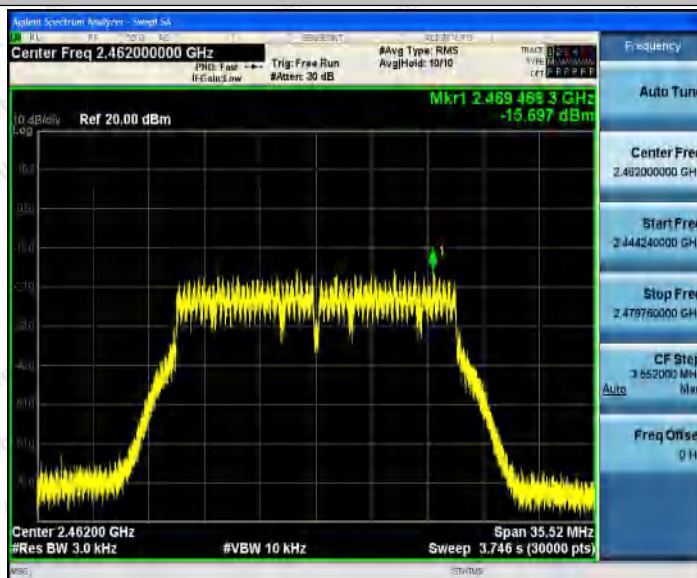
11N20_Ant2_2462
