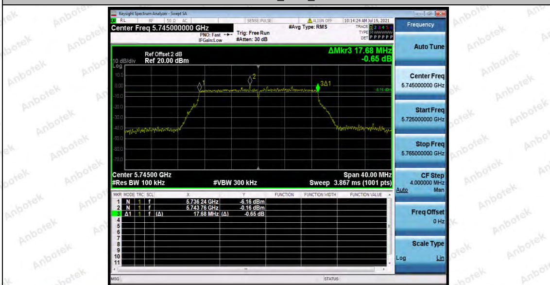
11N20SISO_Ant2_5745
