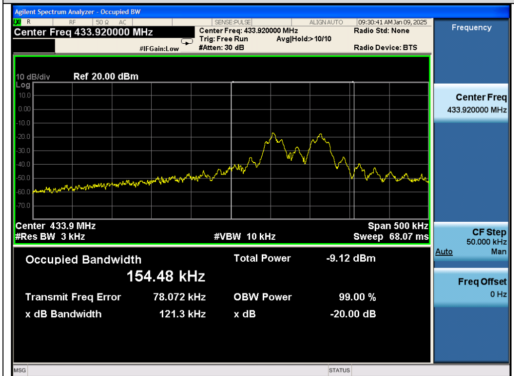
Test_Graph_FSK_433.92MHz_OBW
