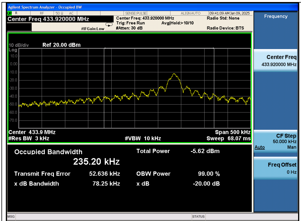
Test_Graph_ASK_433.92MHz_OBW
