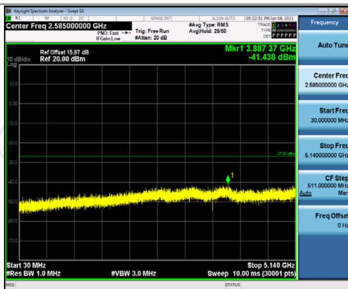
11N40SISO_Ant1_5190_30~5140
