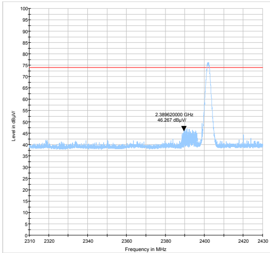
BLE -Channel 0: Average
