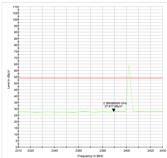
BLE -Channel 0: Average
