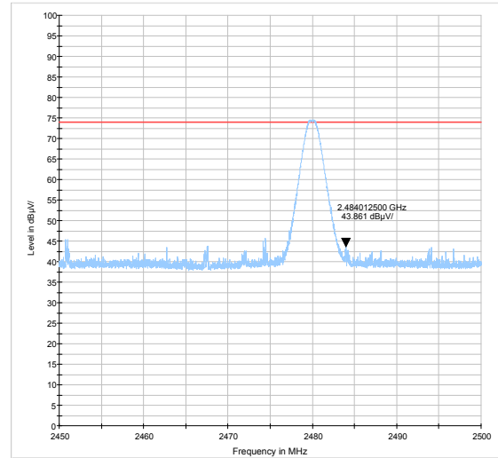
BLE -Channel 39: Average
