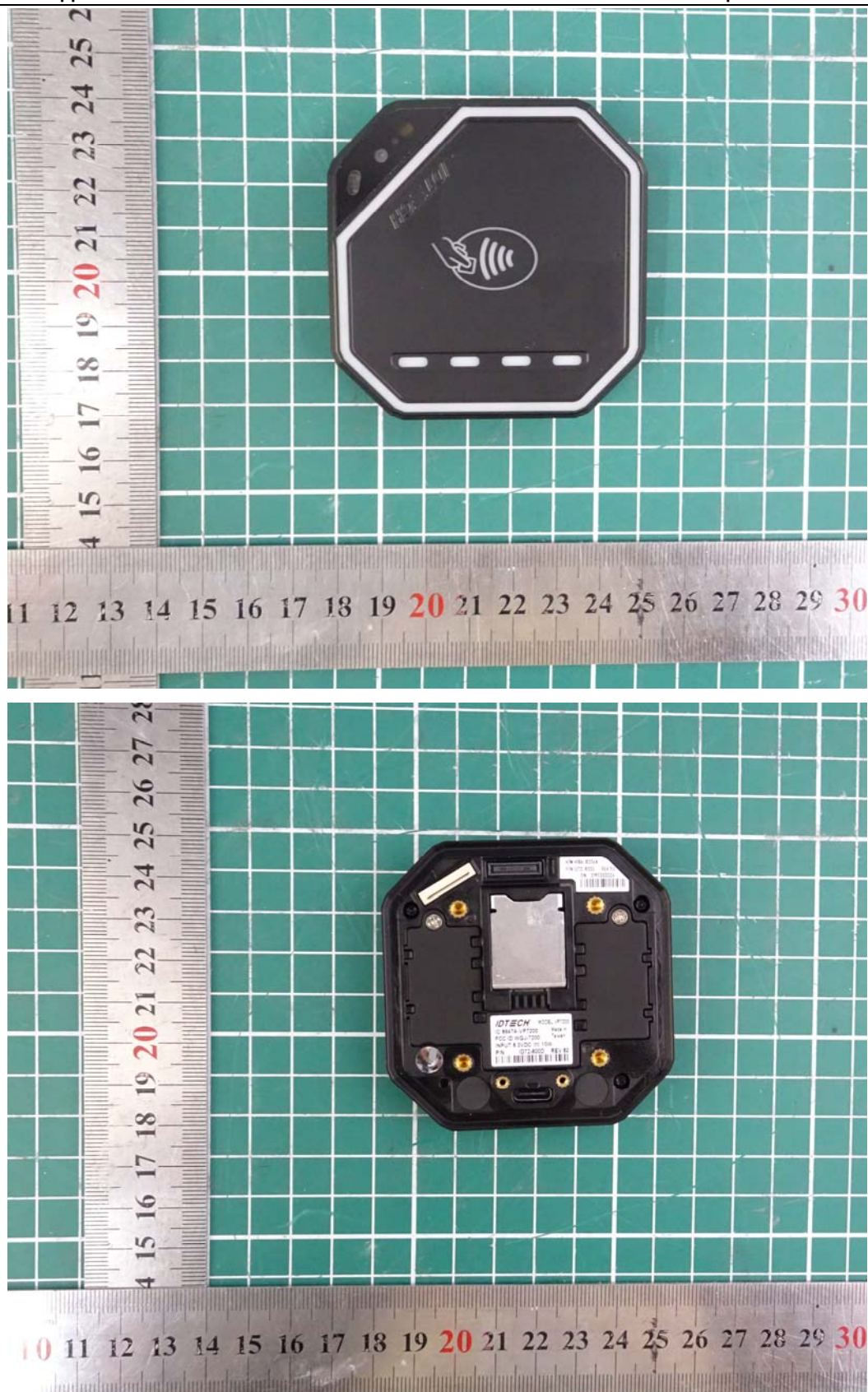
ID72-800; ID72-800D
