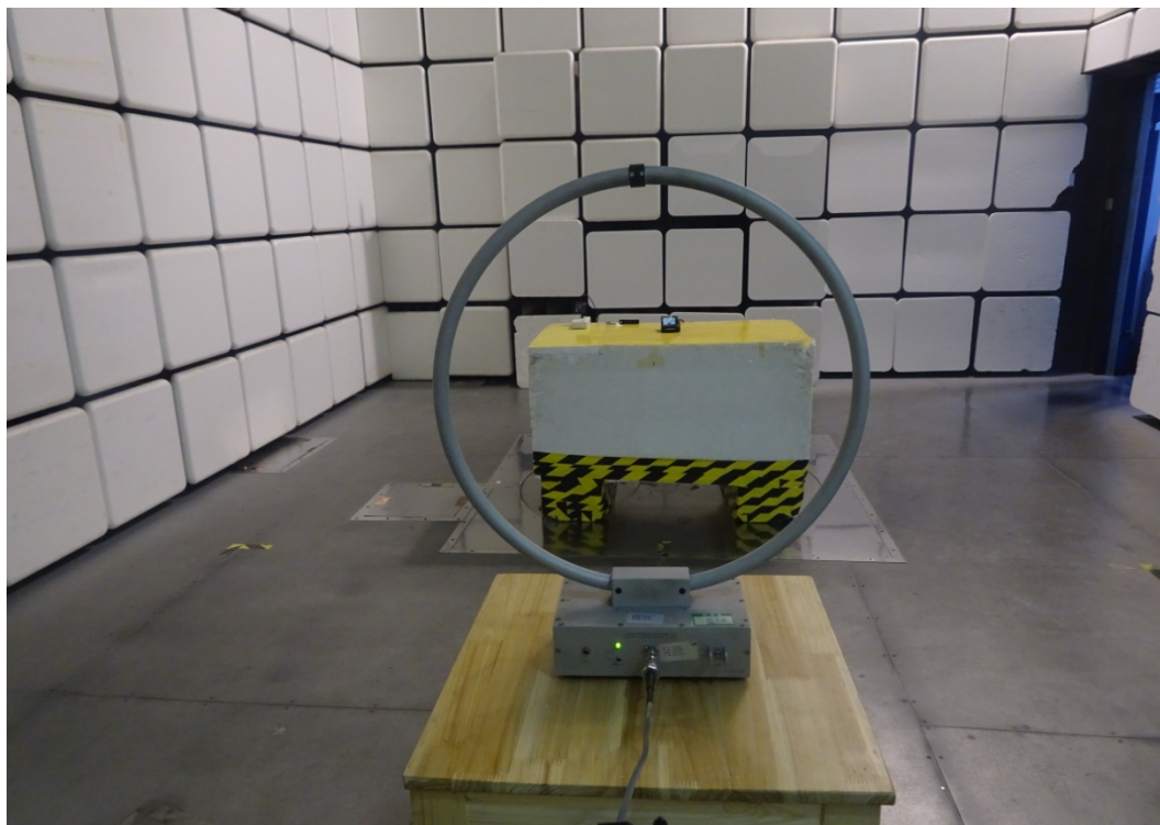
9kHz - 30MHz
