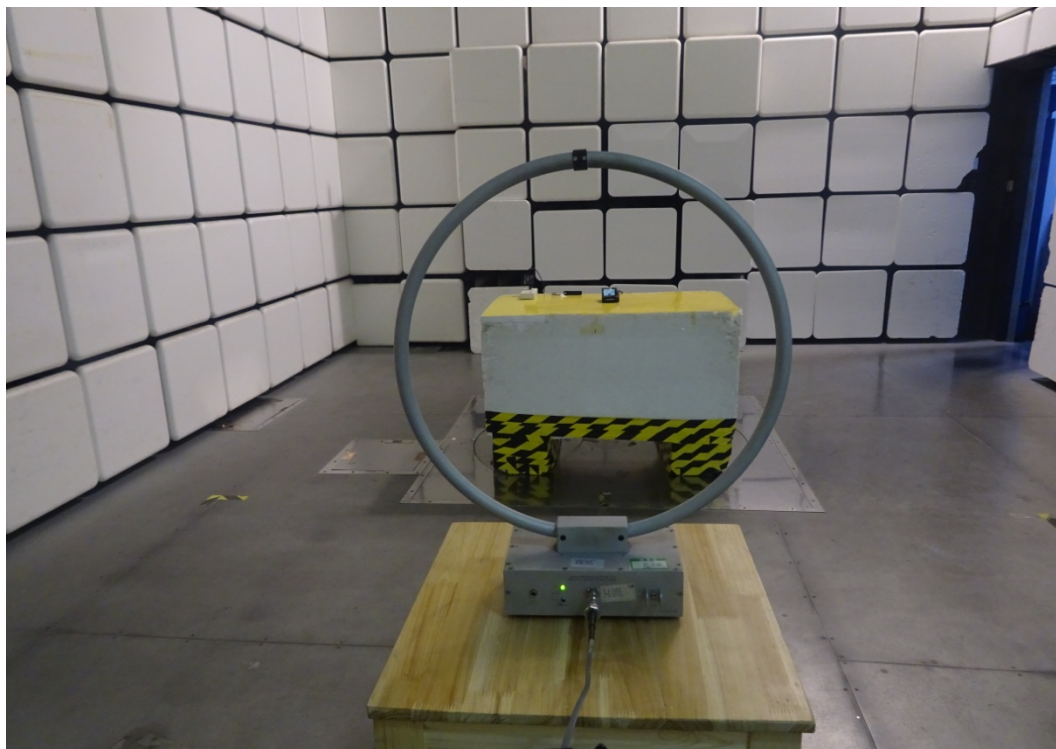
9kHz - 30MHz
